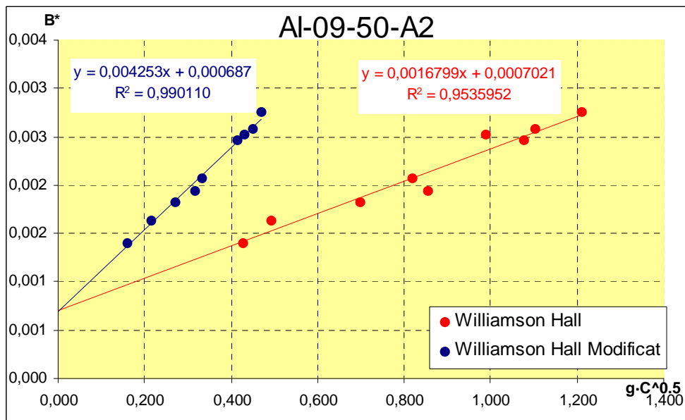
Figura A1.12: resolució gràfica per a l'AI-09-50-A2
