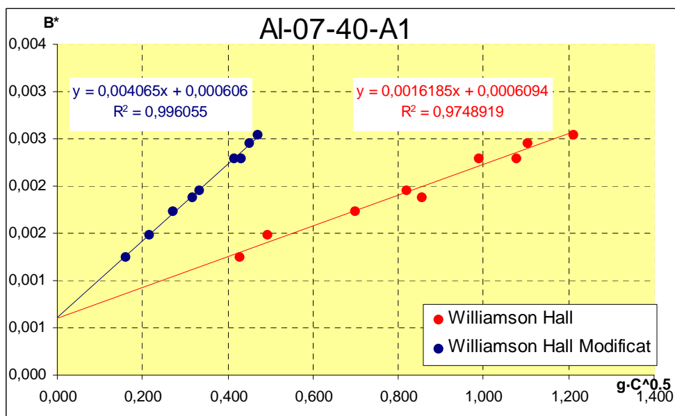
Figura A1.6: resolució gràfica per a l'AI-07-40-A1
