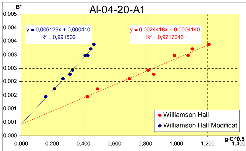
Figura A1.9: resolució gràfica per a l'AI-04-20-A1
