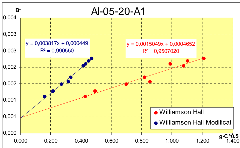
Figura A1.4: resolució gràfica per a l'AI-05-20-A1
