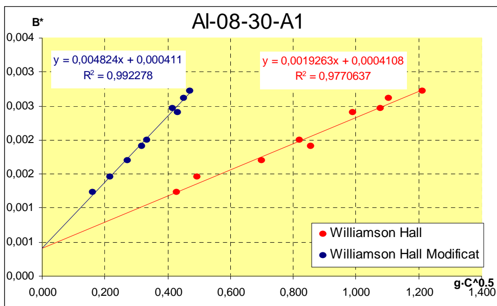
Figura A1.5: resolució gràfica per a l'AI-08-30-A1
