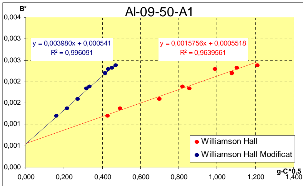
Figura A1.7: resolució gràfica per a l'AI-09-50-A1
