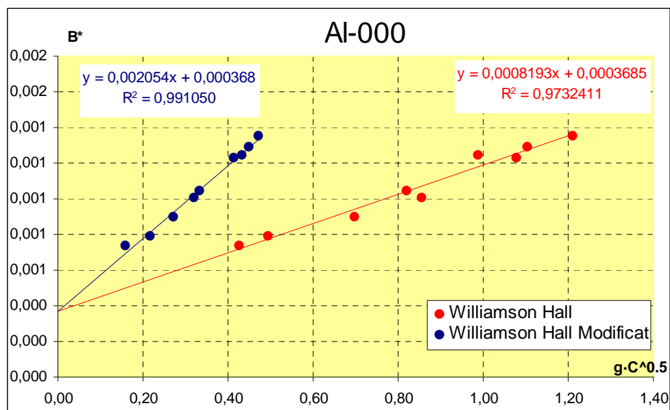
Figura A1.2: resolució gràfica per a l'AI-000
