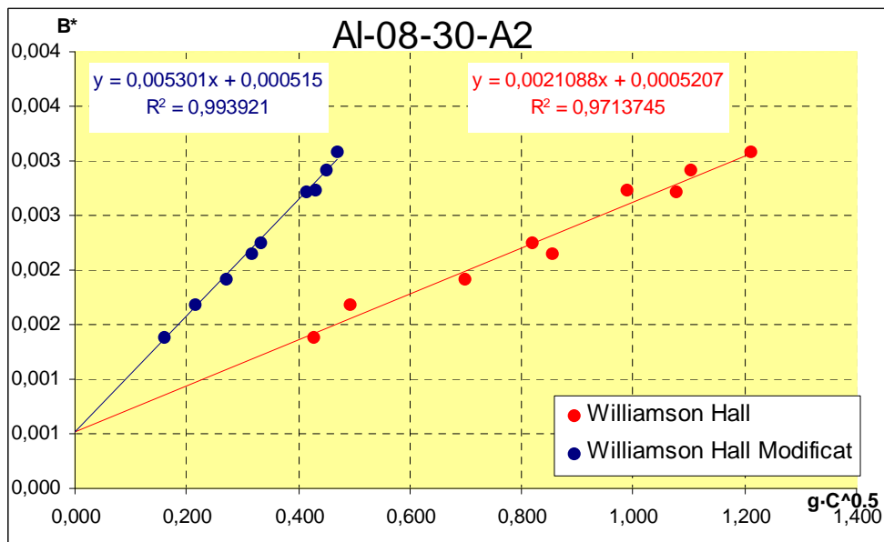
Figura A1.10: resolució gràfica per a l'AI-08-30-A2
