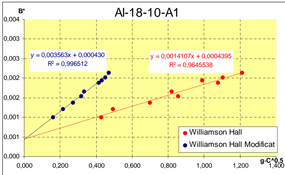
Figura A1.3: resolució gràfica per a l'AI-18-10-A1
