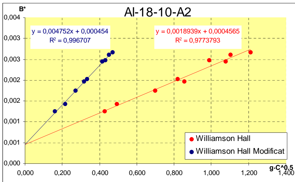
Figura A1.8: resolució gràfica per a l'AI-18-10-A2
