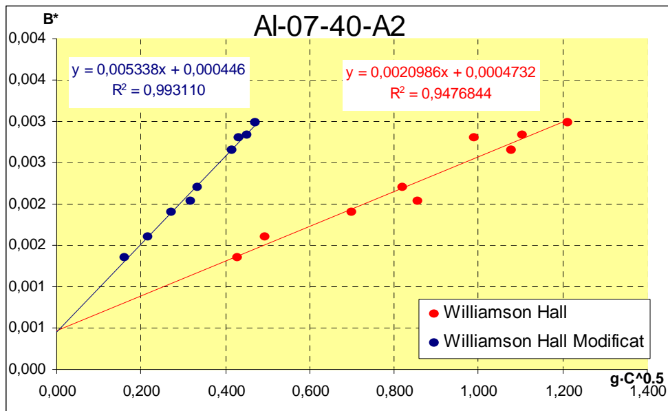
Figura A1.11: resolució gràfica per a l'AI-07-40-A2
