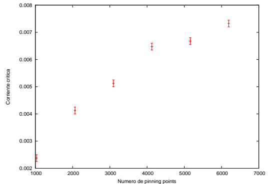
Figura 2: Curva de dependencia de la corriente crítica con el número de pinning points , se puede ver que para N_p \lesssim 4128 el perfil es muy aproximadamente lineal mientras que para N_p mayores la forma de la curva cambia dando lugar a un crecimiento mucho más lento
