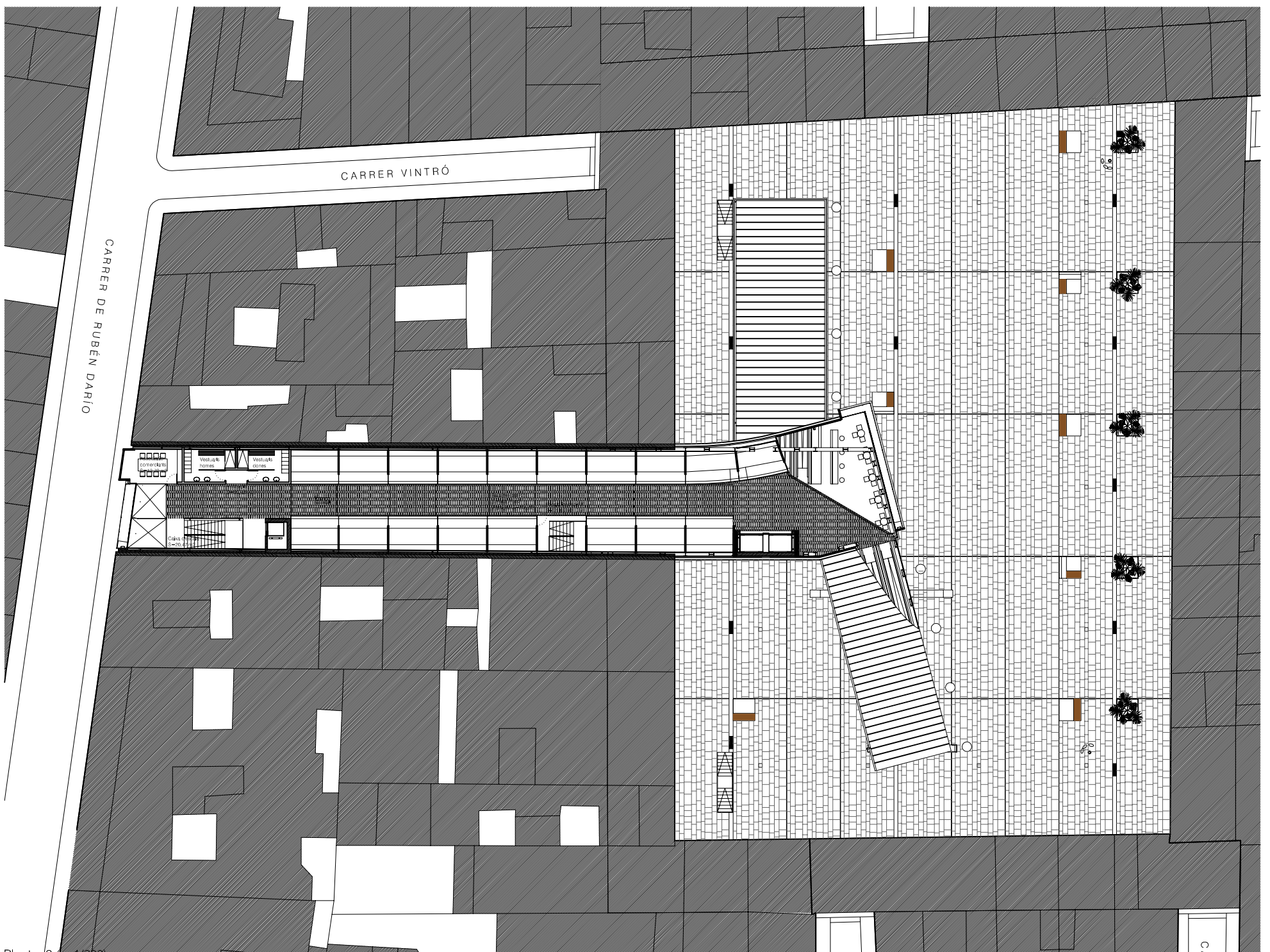
Planta 2 (e: 1/200)
