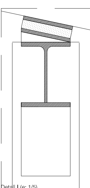
Detall I (e: 1/5)
