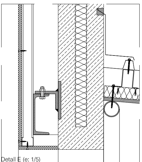
Detall E (e: 1/5)
