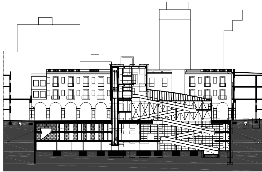
Referència detalls constructius secció 2
