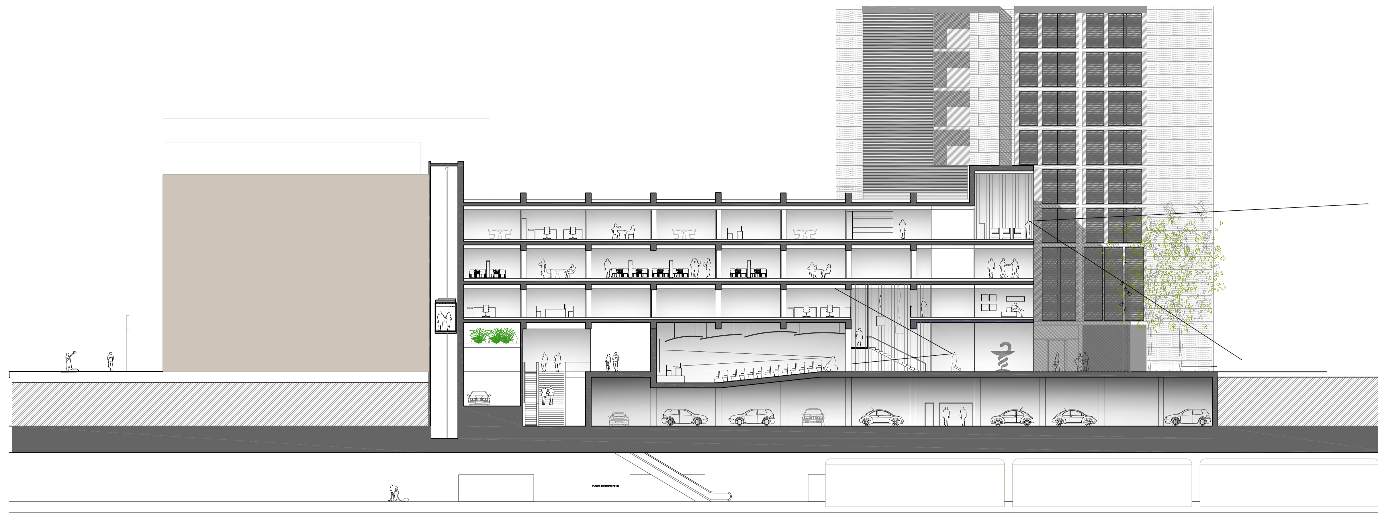
SECCIÓ LONGITUDINAL COL.LEGI
