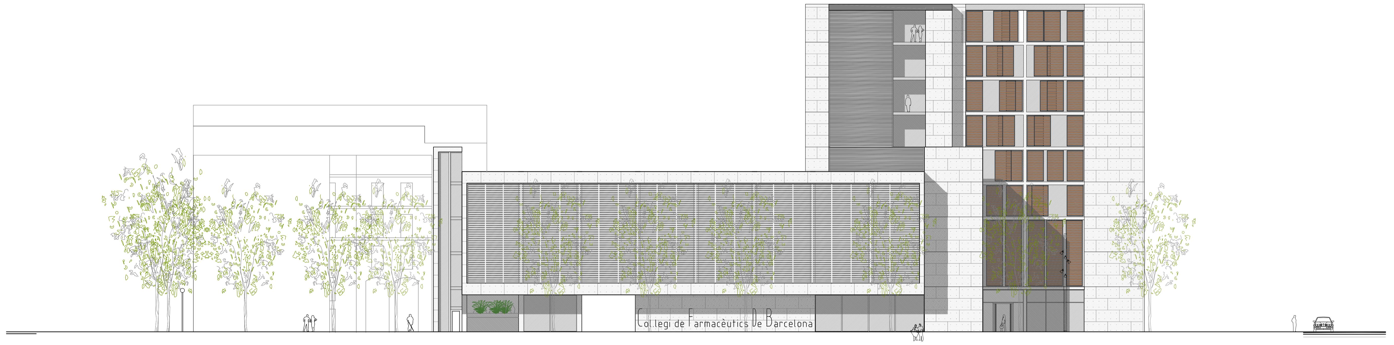
ALÇAT SUD-EST e 1/200 0 2 4
