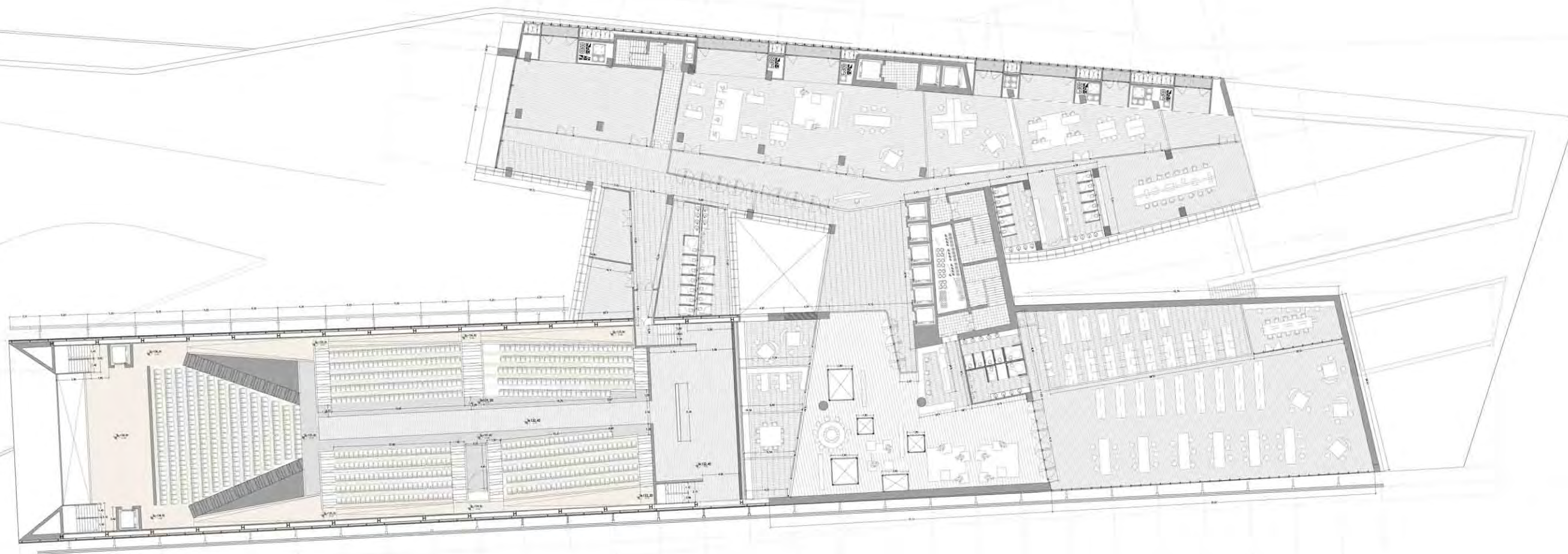
Planta Cinquena, Biblioteca, Dependències de l'auditori, direcció i administració del conjunt
