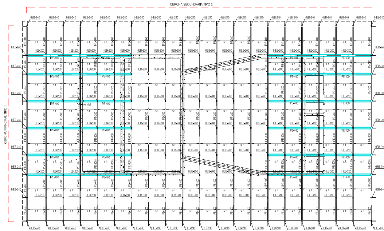
PLANTA CUBIERTA
