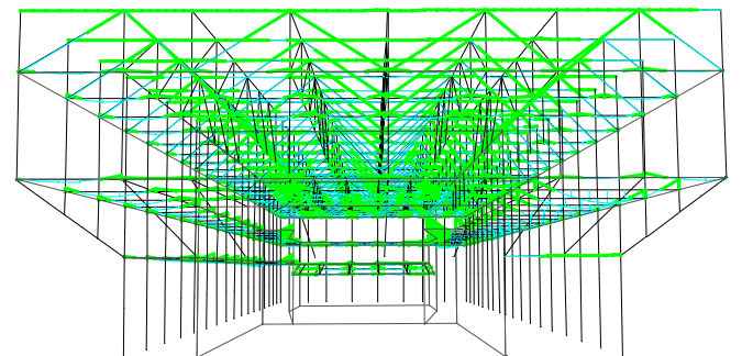
DIAGRAMA DE MOMENTOS FLECTORES
