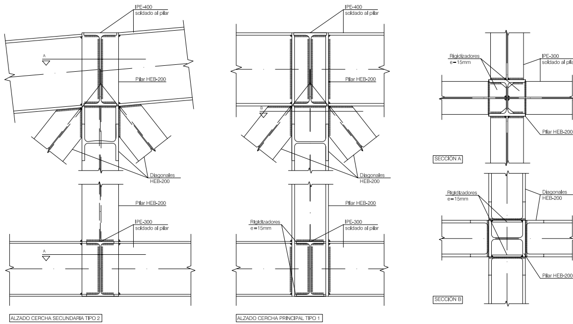
DETALLE NUDO ENCUENTRO CERCHA PRINCIPAL TIPO 1 CON CERCHA SECUNDARIA TIPO 2
