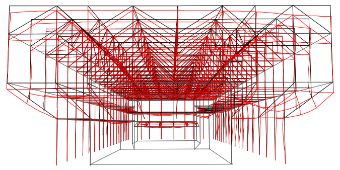
DIAGRAMA DE DEFORMACIONES
