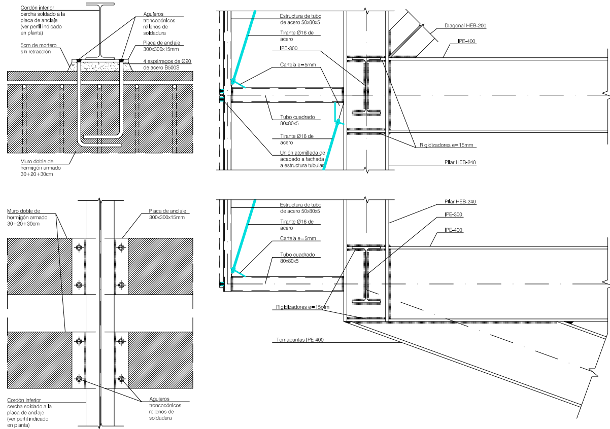
DETALLE UNIÓN CORDÓN INFERIOR CERCHA-MURO
