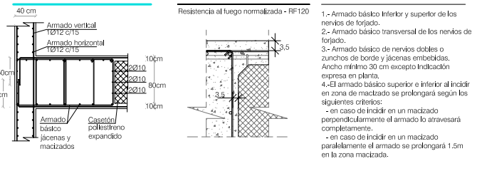
DETALLE DEL FORJADO LOSA NERVADA TIPO SANDWICH
