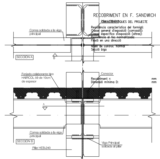
DETALLE UNIÓN PILAR-VIGA-CORREA
