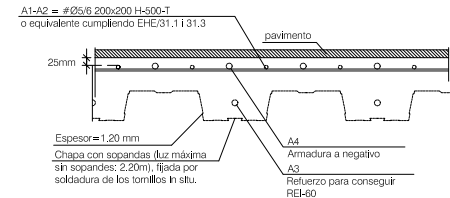
DETALLE DEL FORJADO COLABORANTE
