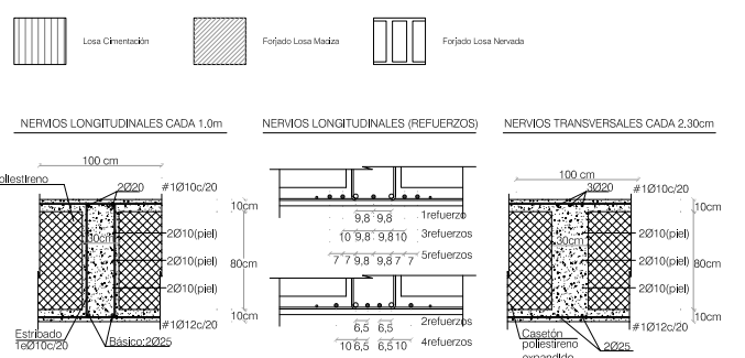
ENCUENTRO MURO-MAQIZADO
