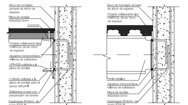
DETALLE UNIÓN DE ESTRUCTURA METÁLICA A MUROS DE HORMIGÓN
