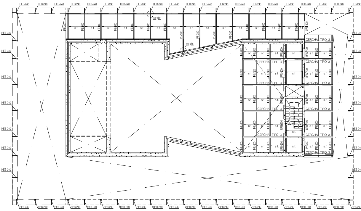
PLANTA PRIMERA
