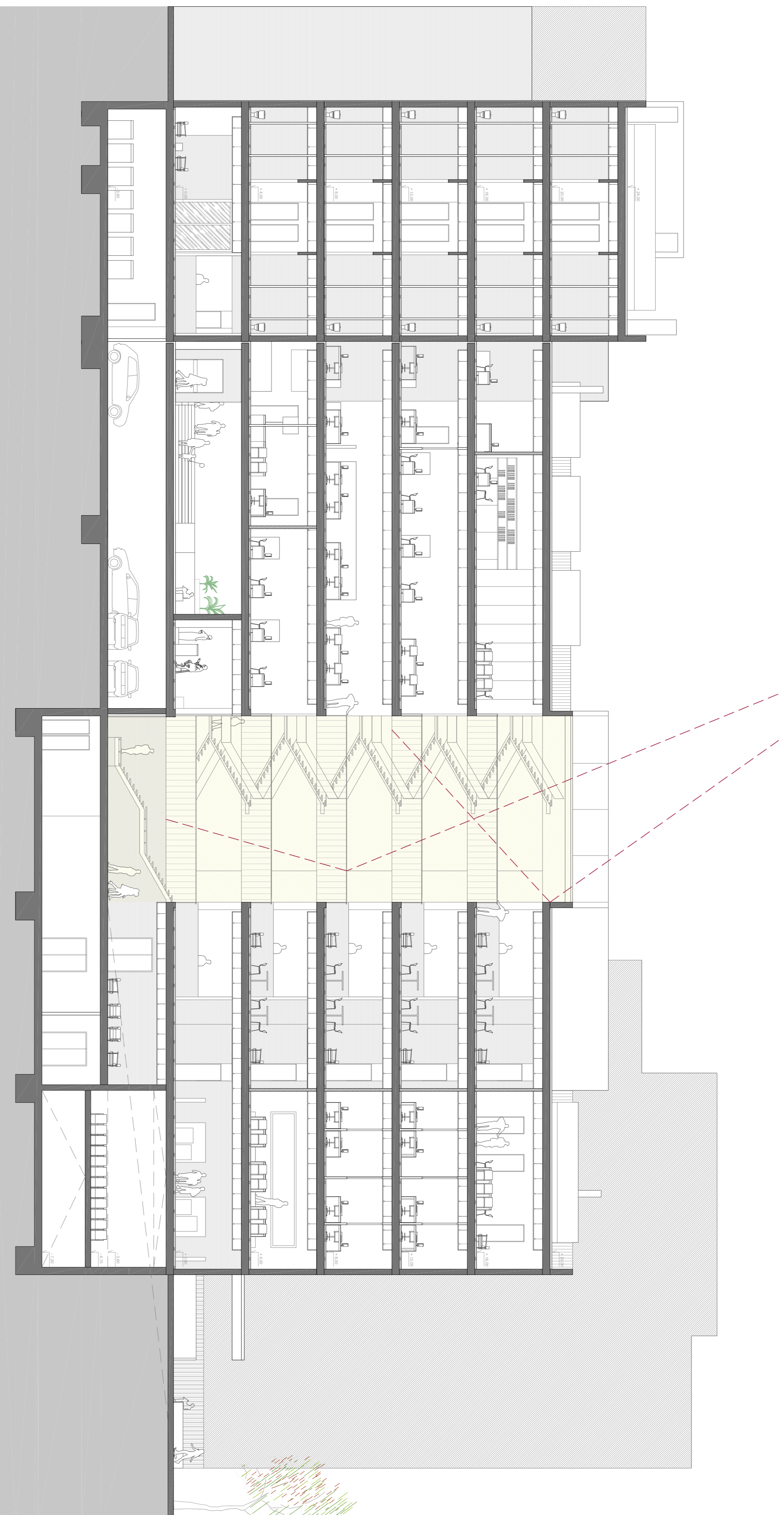
SECCIÓ LONGITUDINAL_S12
