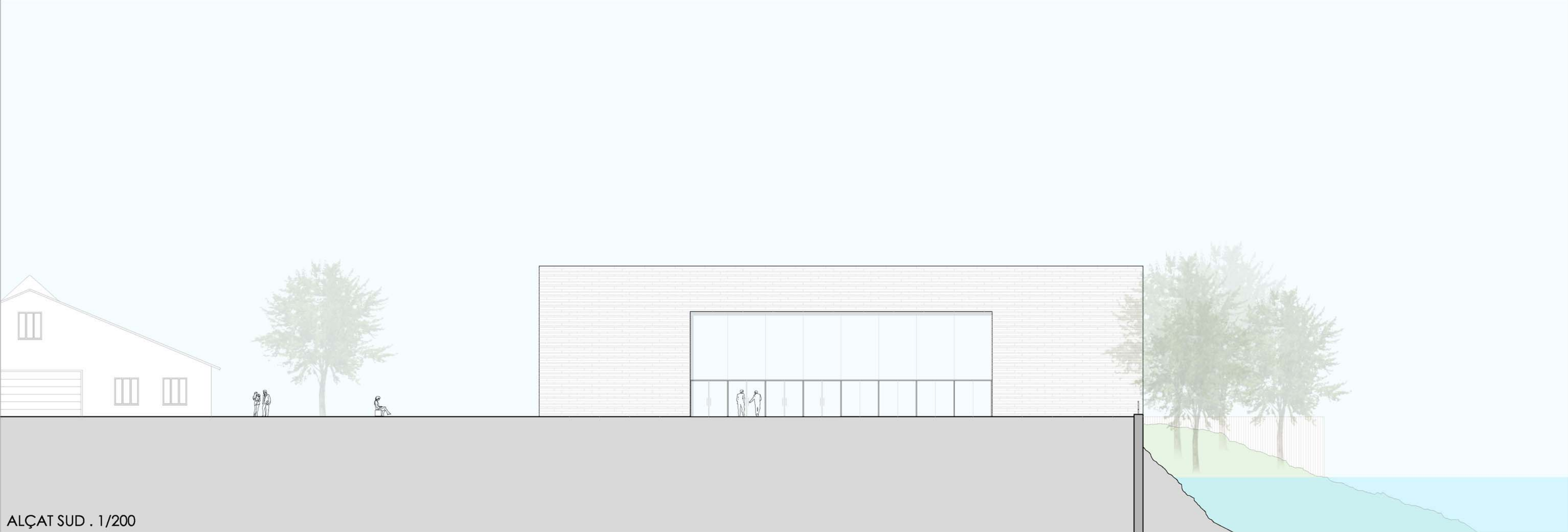
ALÇAT SUD . 1/200
