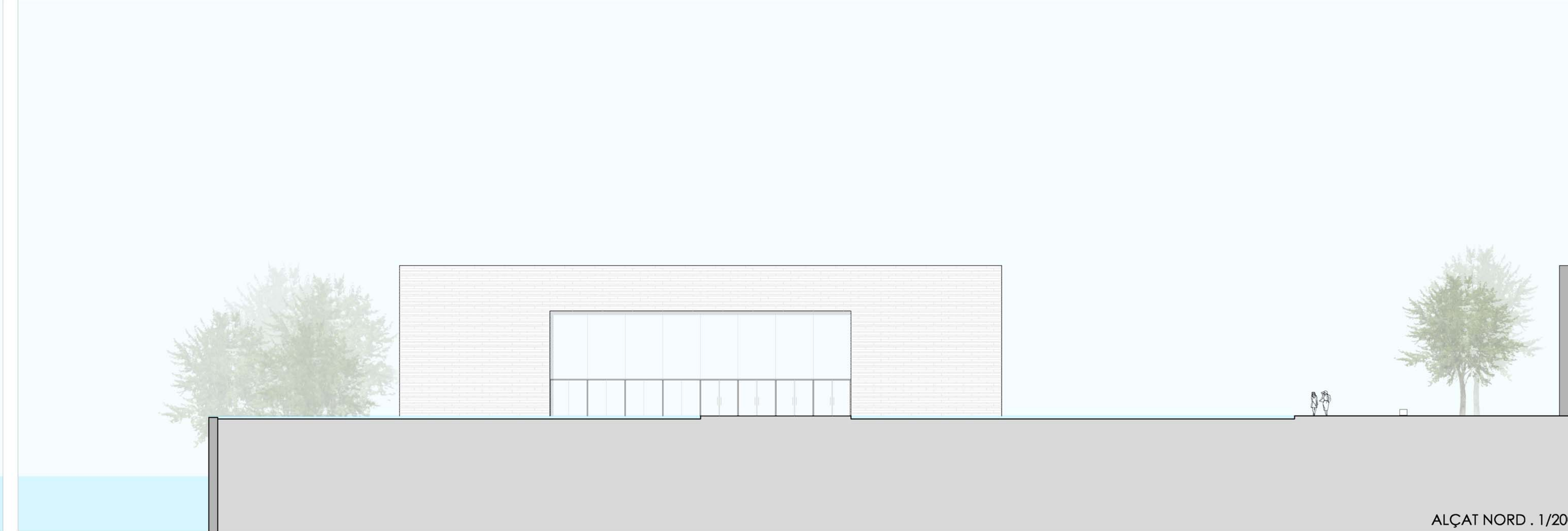
ALÇAT NORD . 1/200
