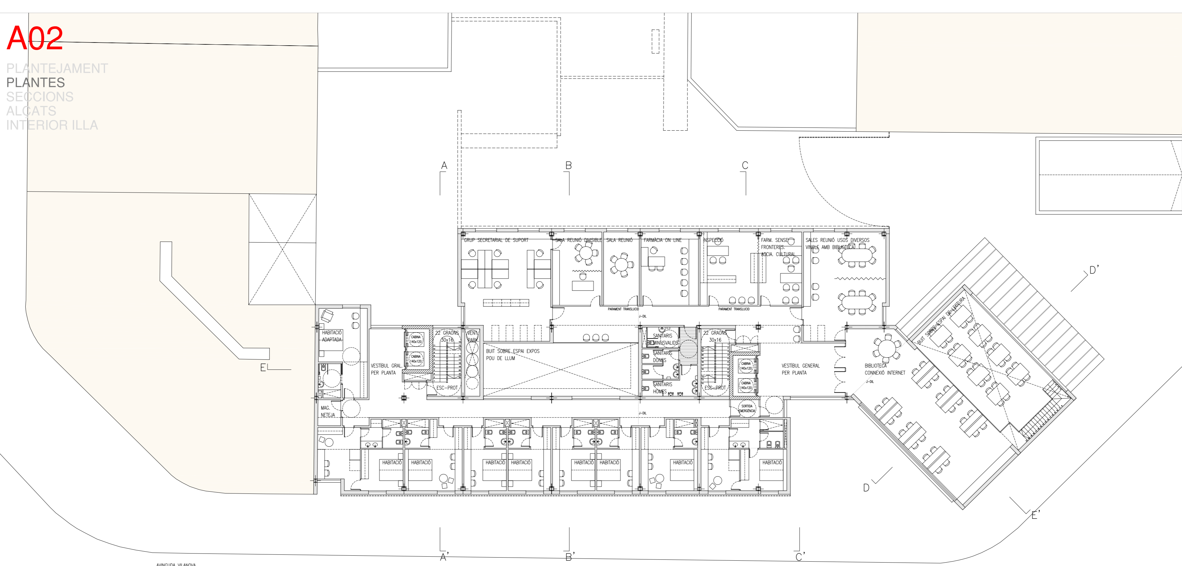
PLANTA TERCER PIS COL·LEGI+HOTEL SUP. CONSTRUÏDA 1113,11m2 COTA GENERAL +11,40
