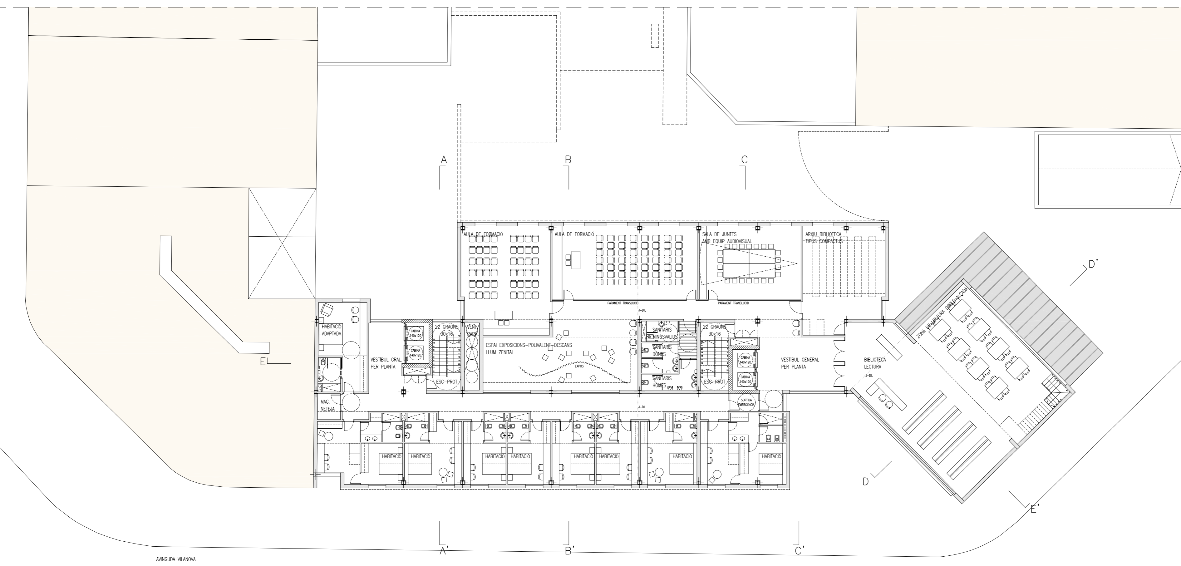
PLANTA SEGON PIS COL·LEGI+HOTEL SUP. CONSTRUÏDA 1113,11m2 COTA GENERAL +7,90
