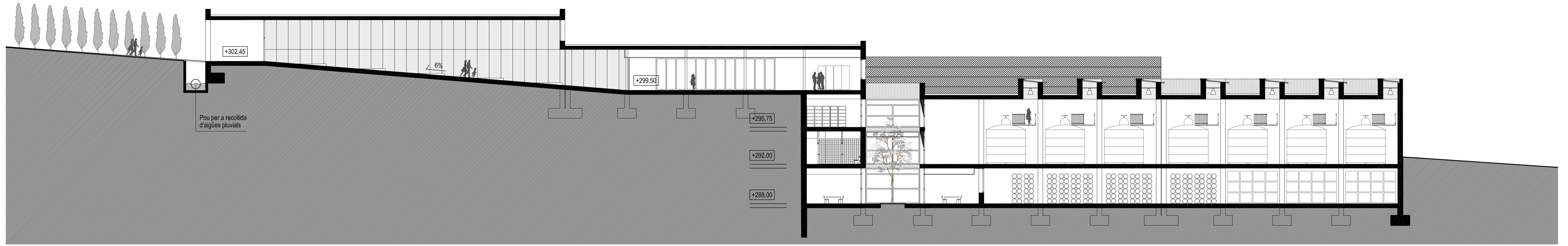
Secció Longitudinal 3
