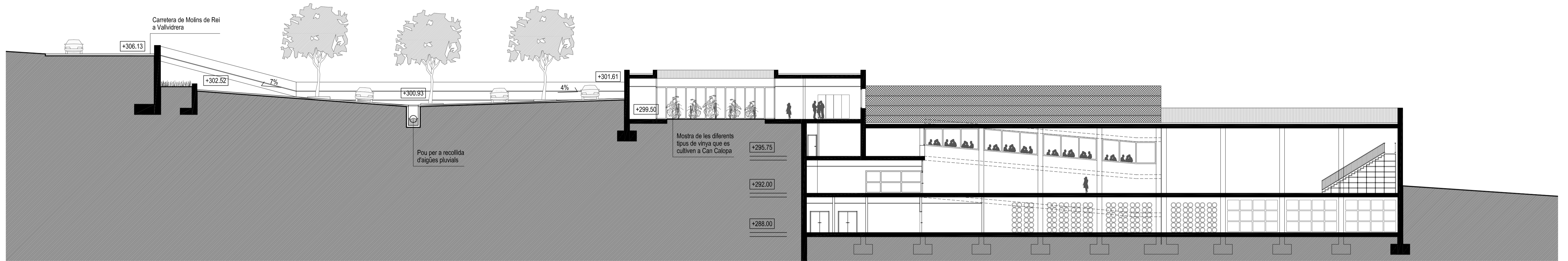
Secció Longitudinal 4
