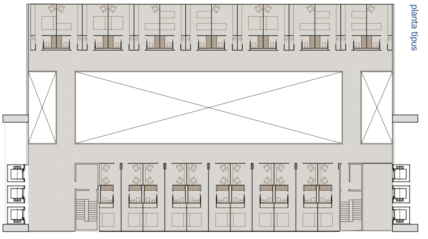
planta terrassa
