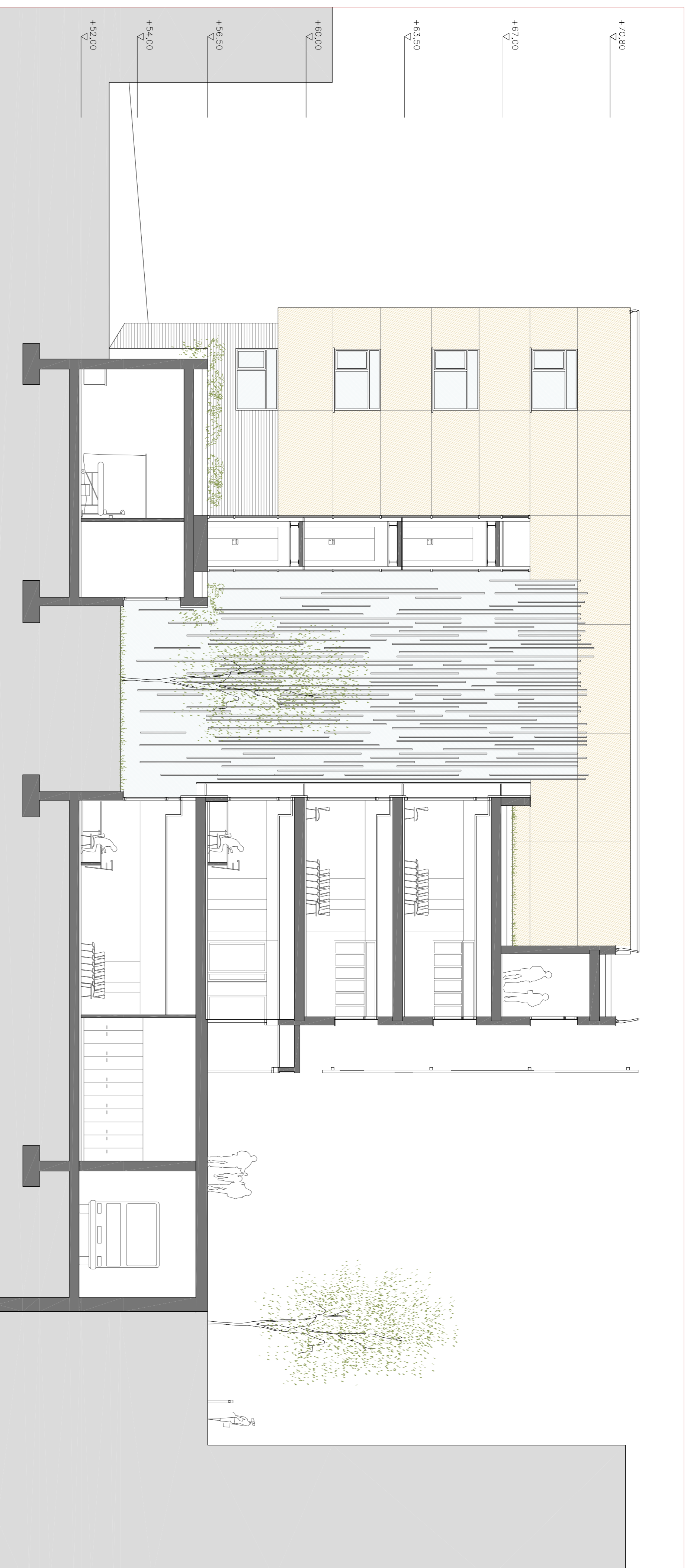
1. Secció Longitudinal bloc Sud.
