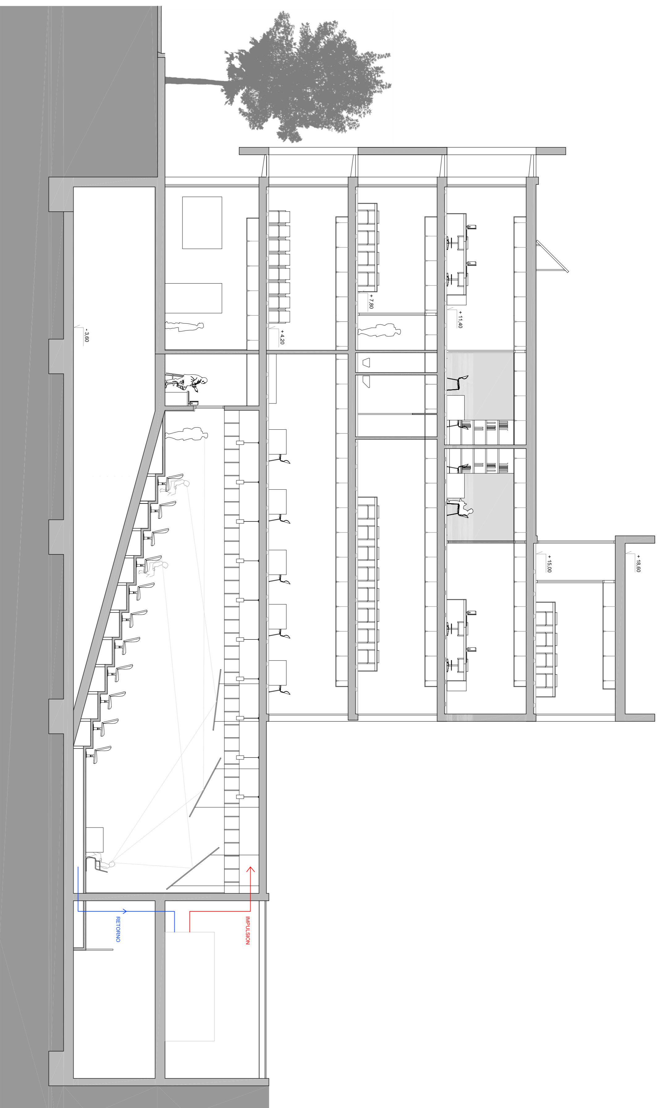
Sección ST3
