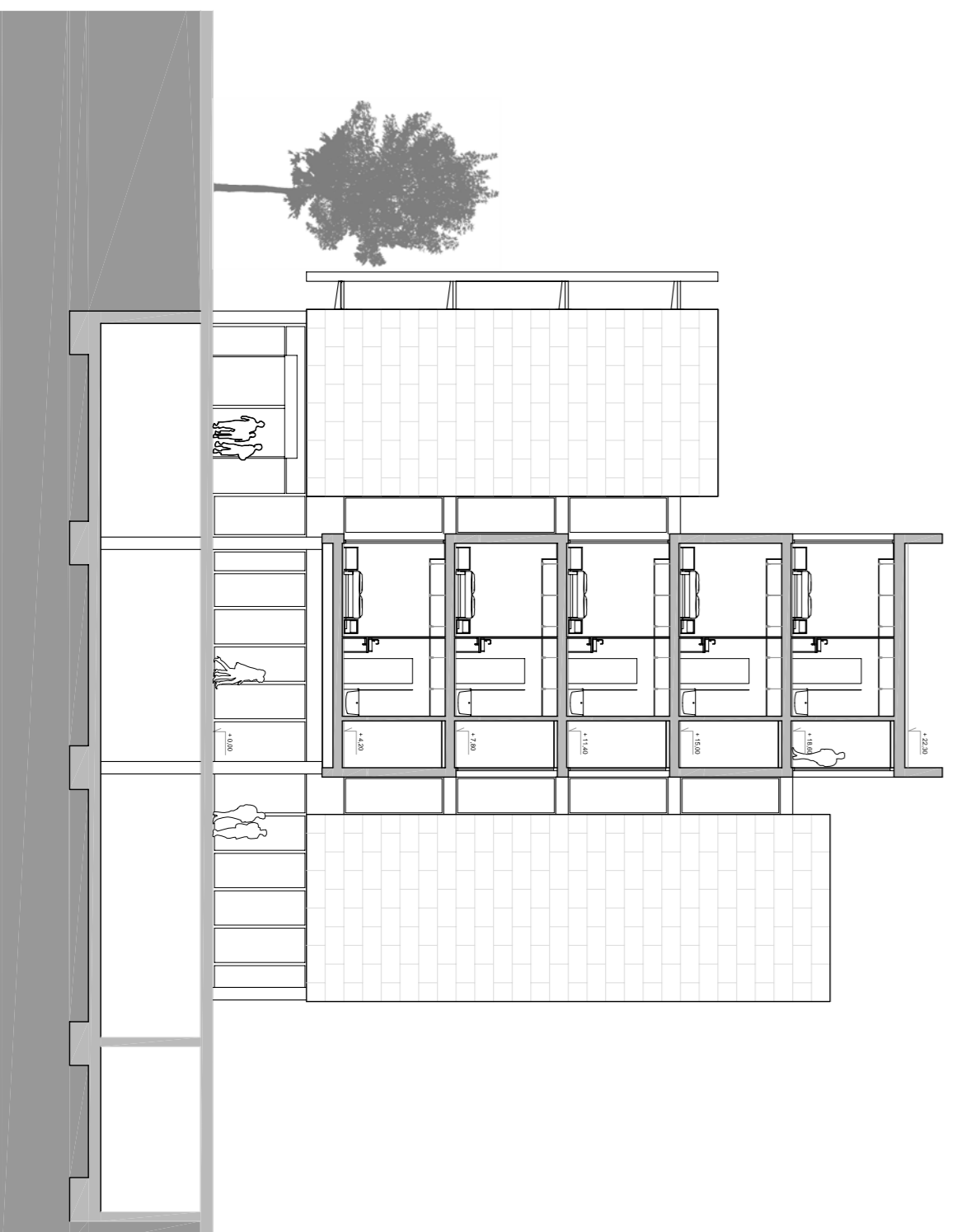
Sección ST1
