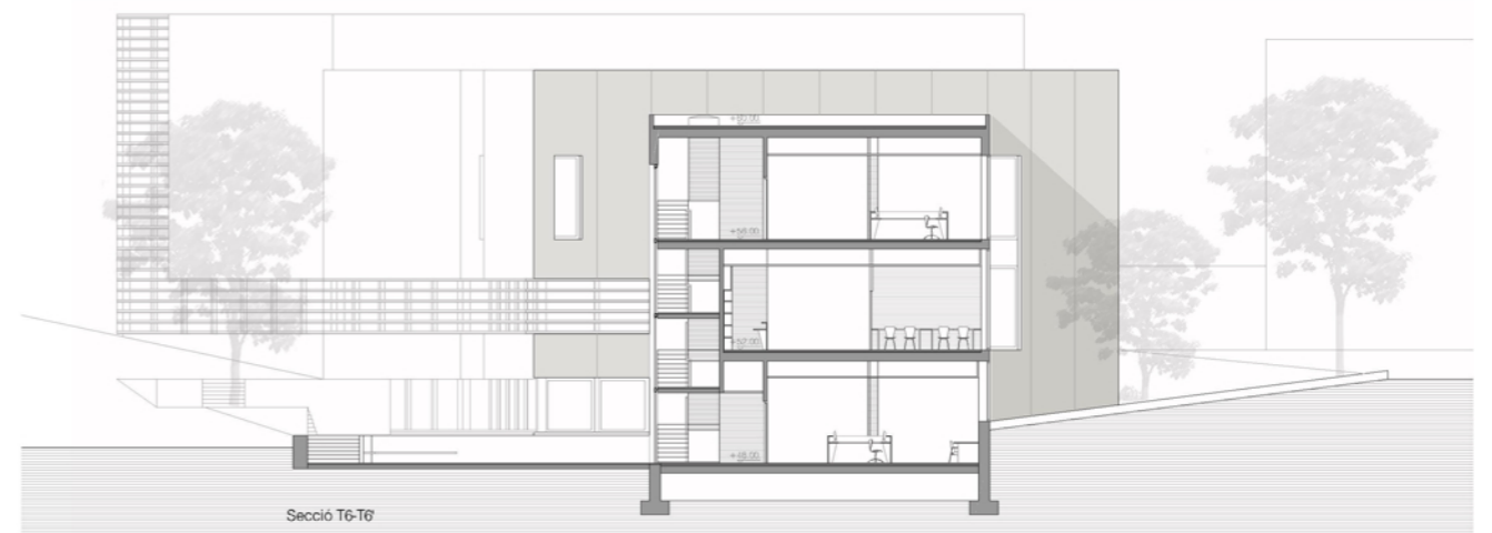
Secció T6-T6''
