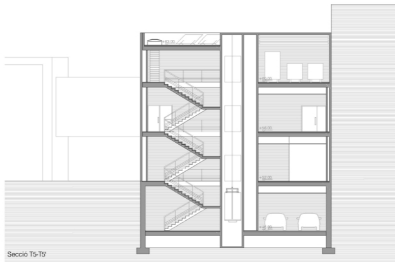
Secció T5-T5''
