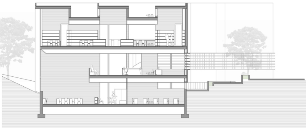
Secció transversal T2-T2'
