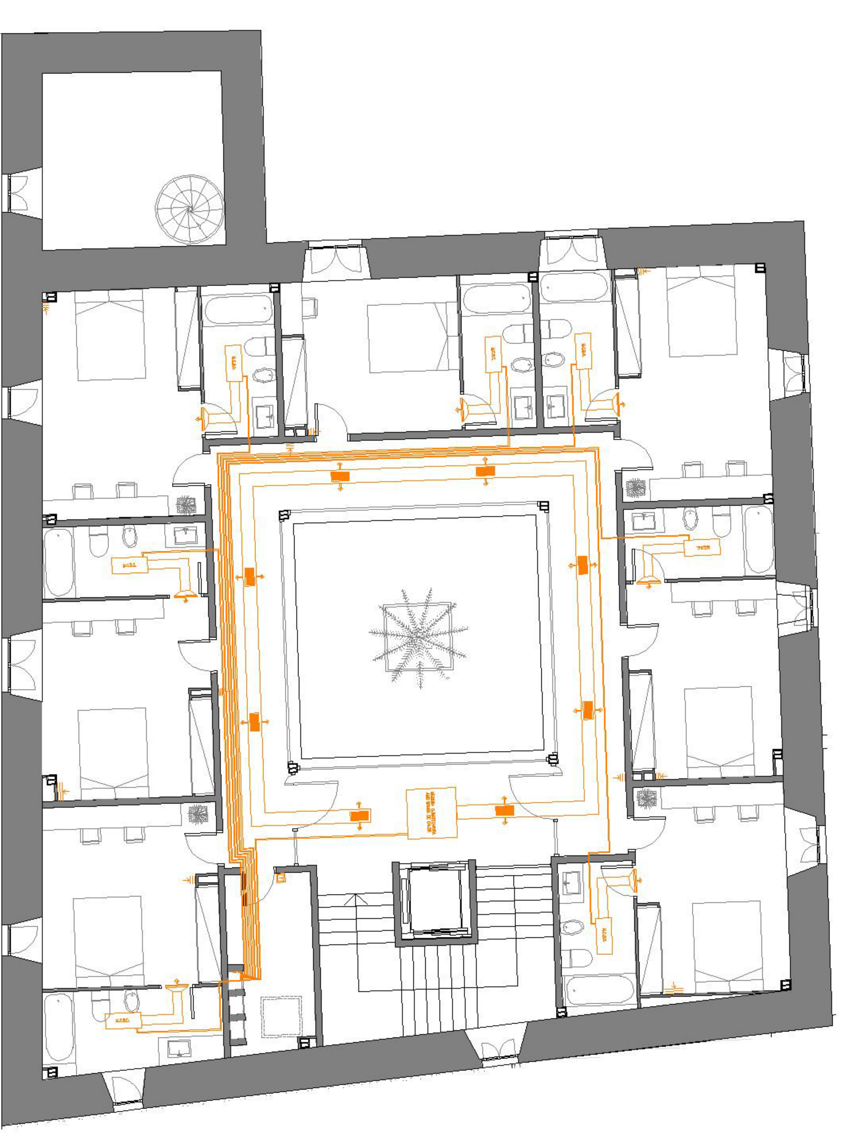
PLANTA SEGONA _CLIMATITZACIÓ_ E:1/100
