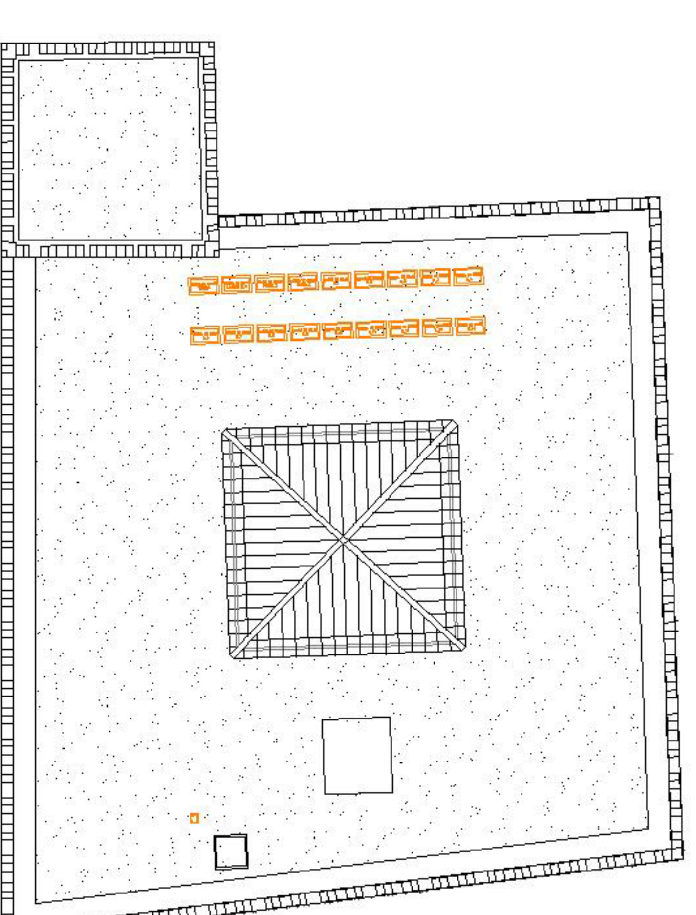
PLANTA COBERTA _CLIMATITZACIÓ_ E:1/200
