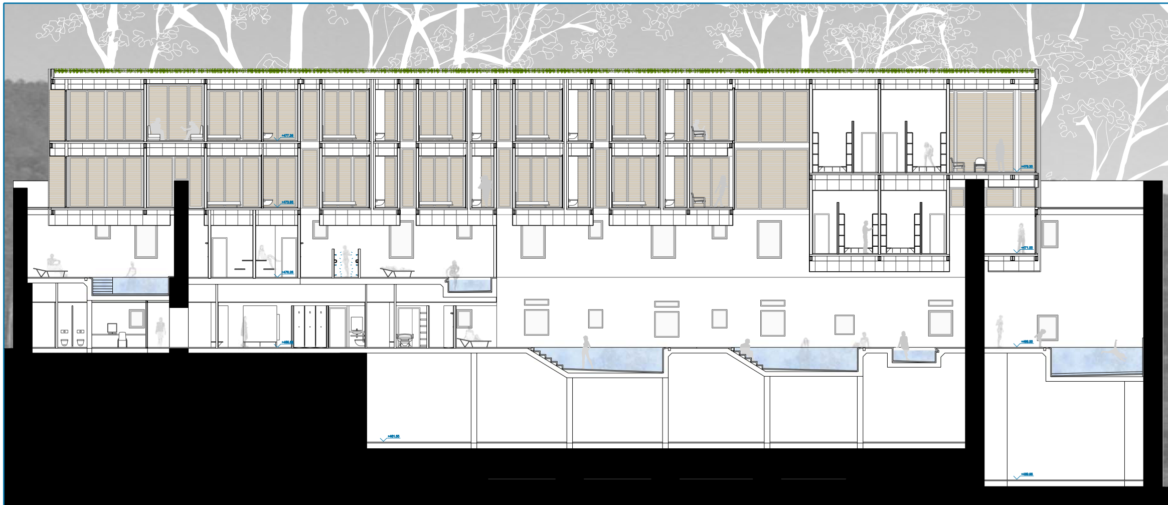
SECCIÓ 6-6', E:1/100
