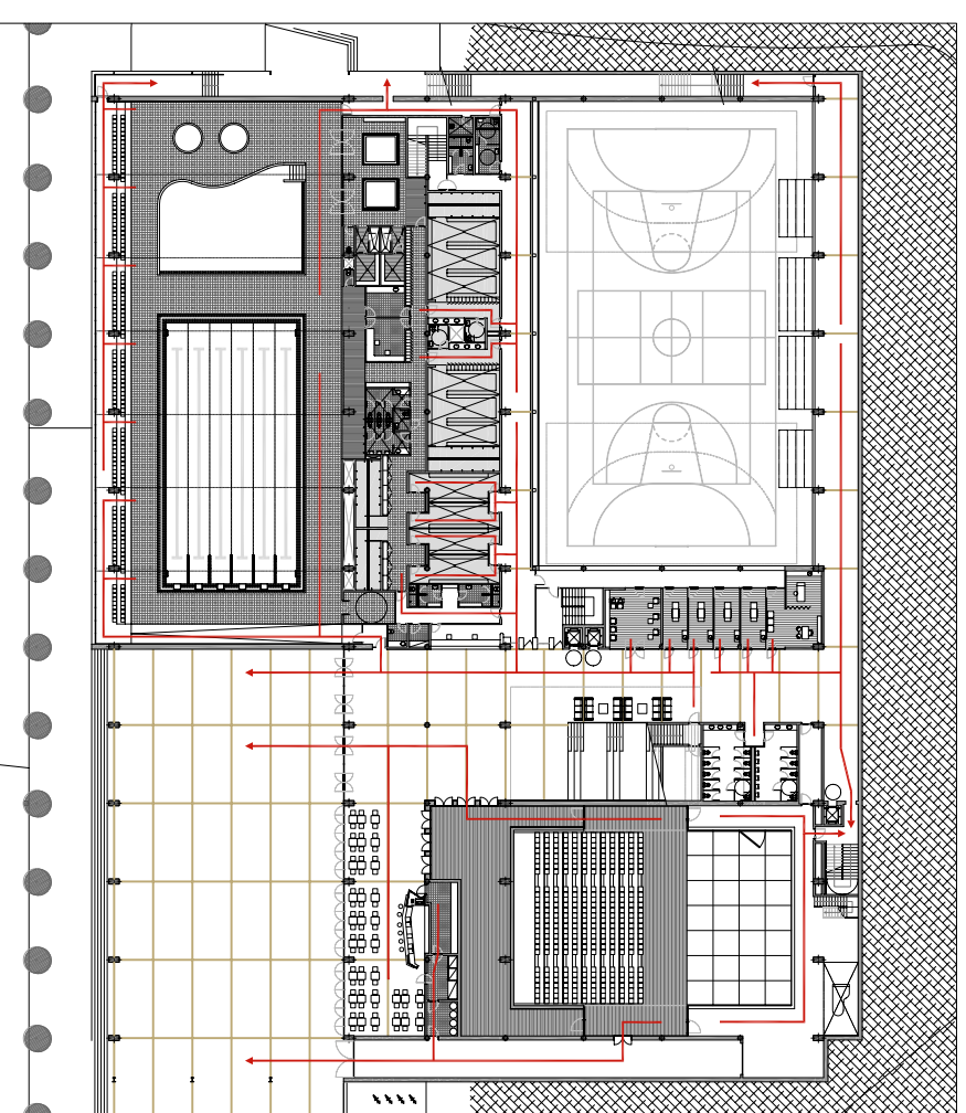
nivell 0 (+74,00)
