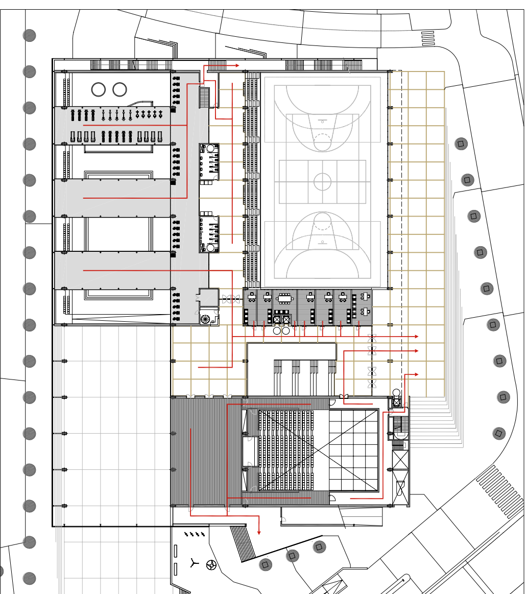
nivell +1 (+78,00)
