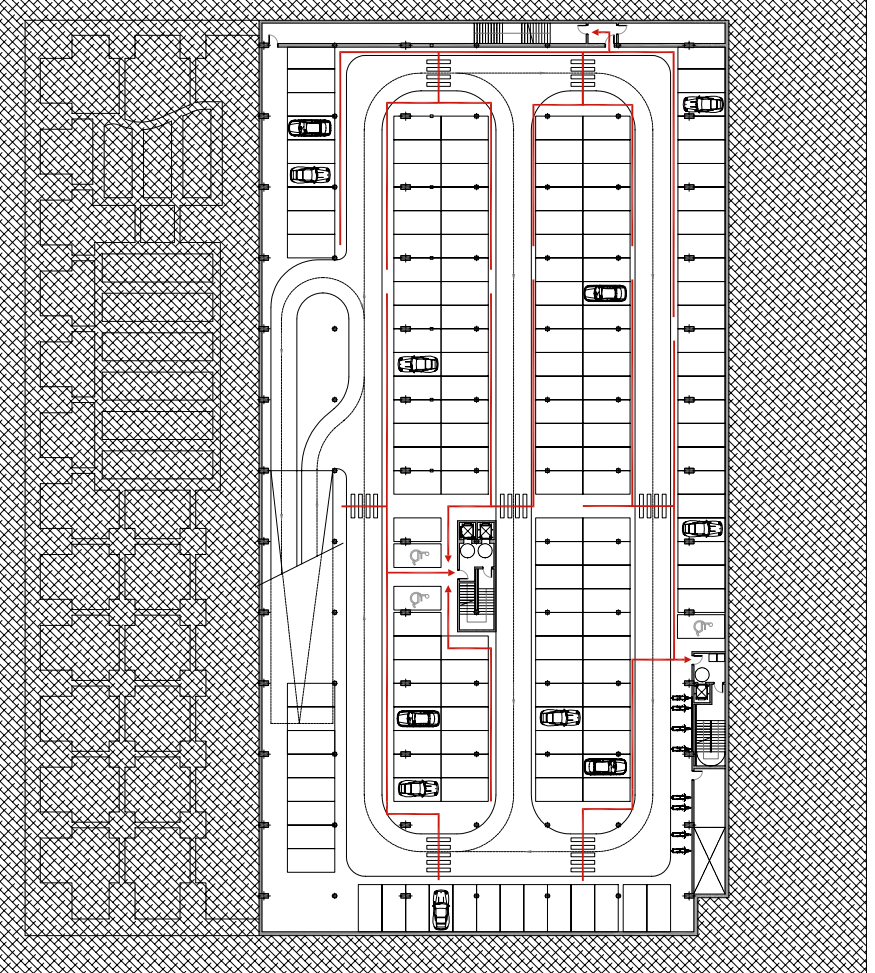
nivell -2 (+66,50)
