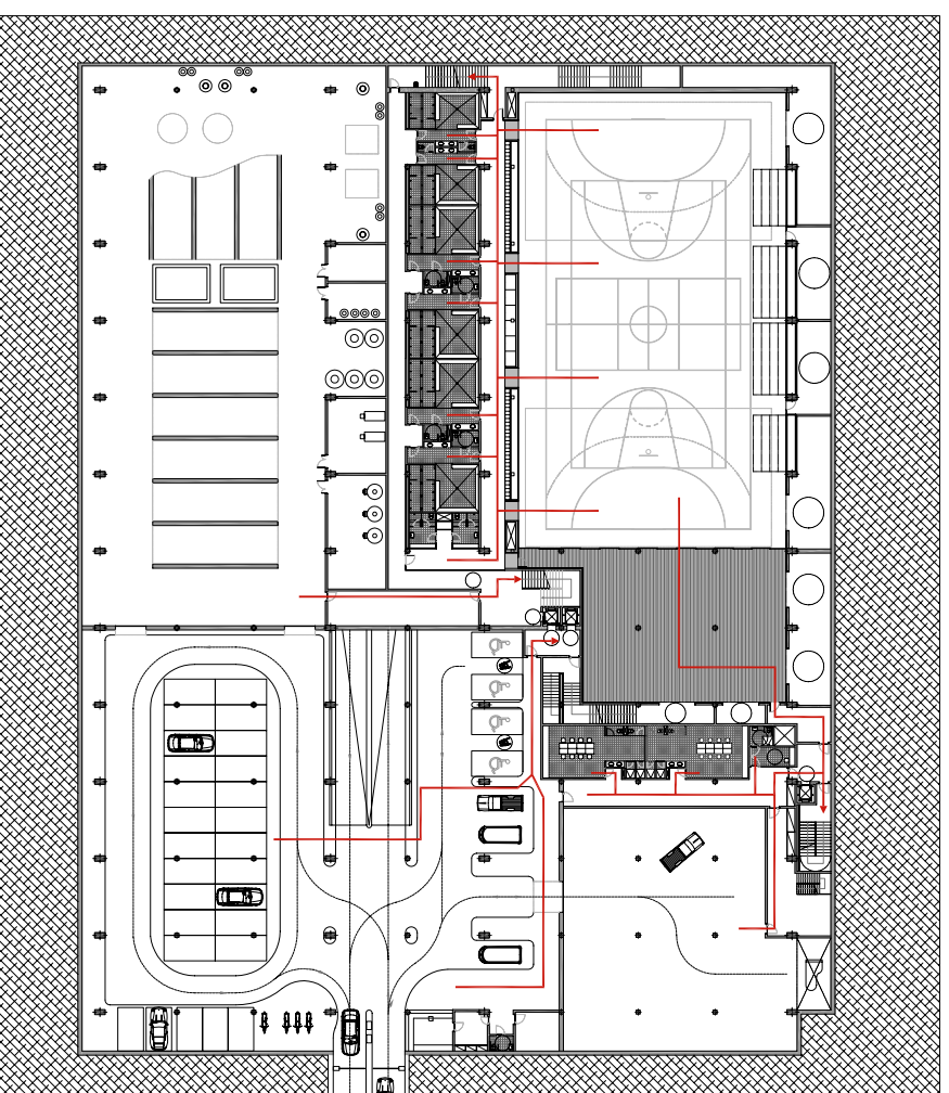
nivell -1 (+70,00)
