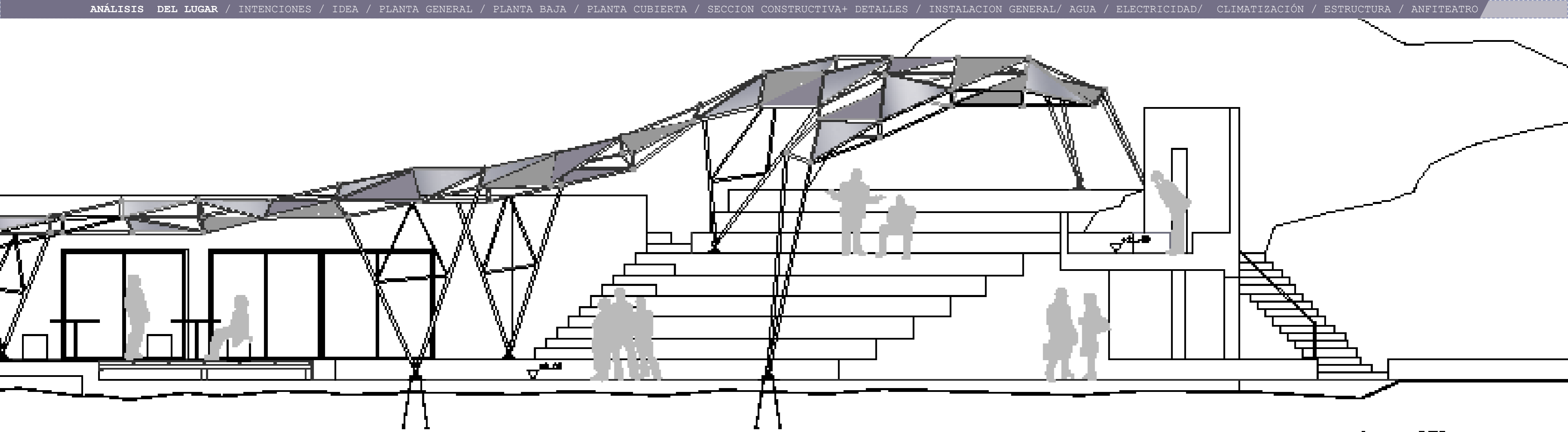
seccion sur. 1/50
