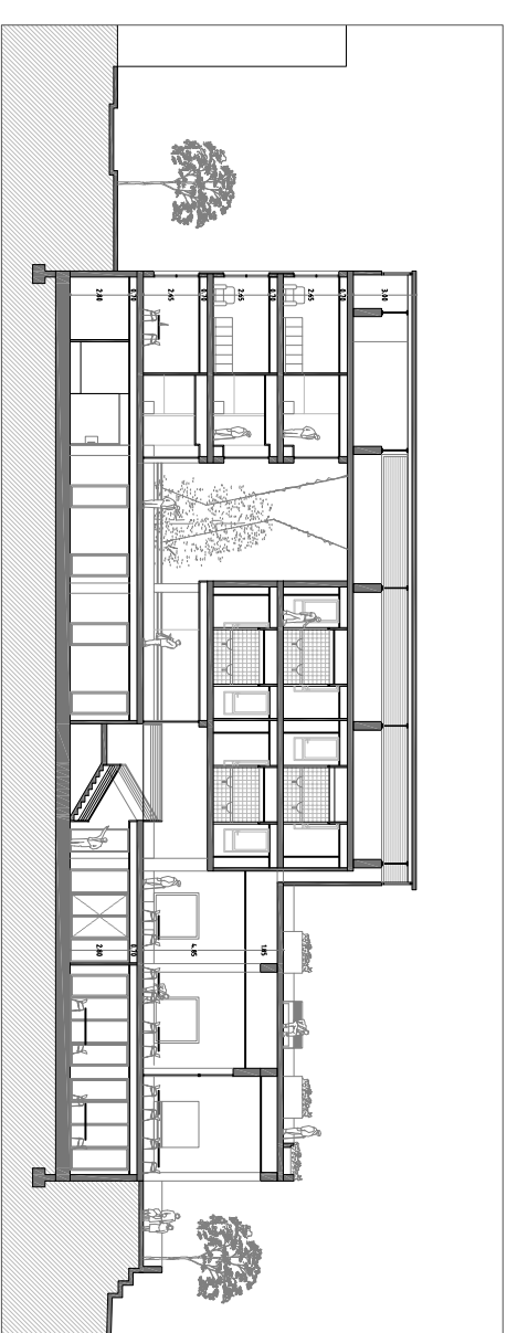
SECCIÓ TRANSVERSAL F
