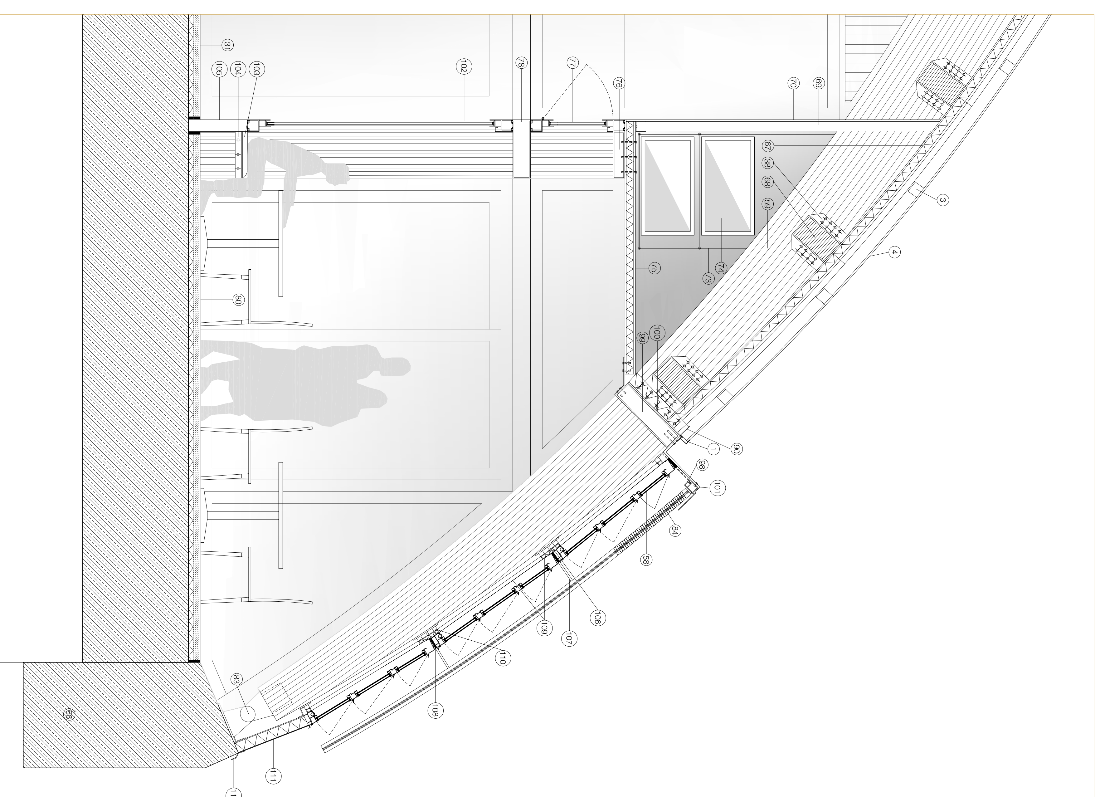
SECCIO F-F ESC:1/20
