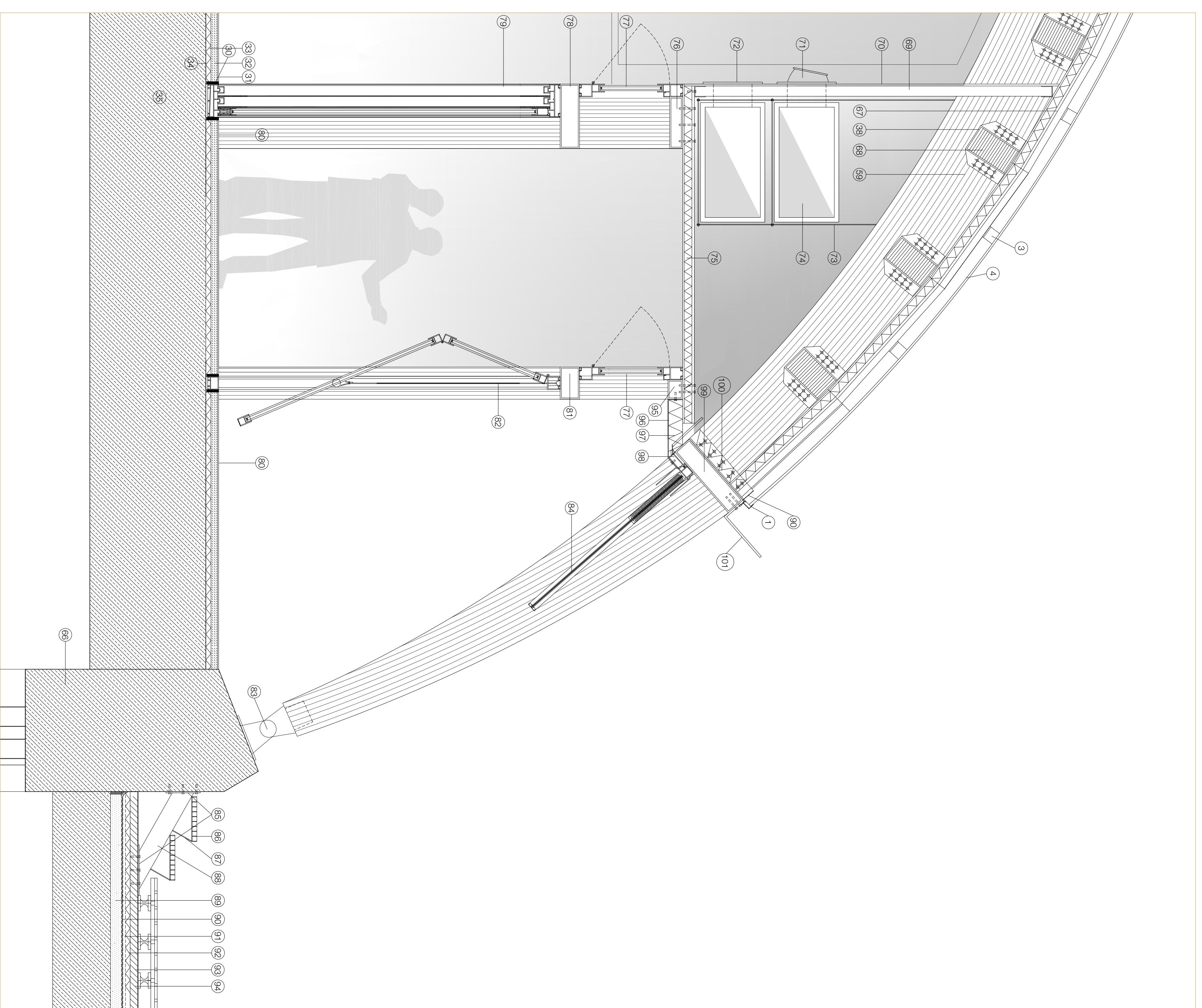
SECCIO E-E ESC:1/20
