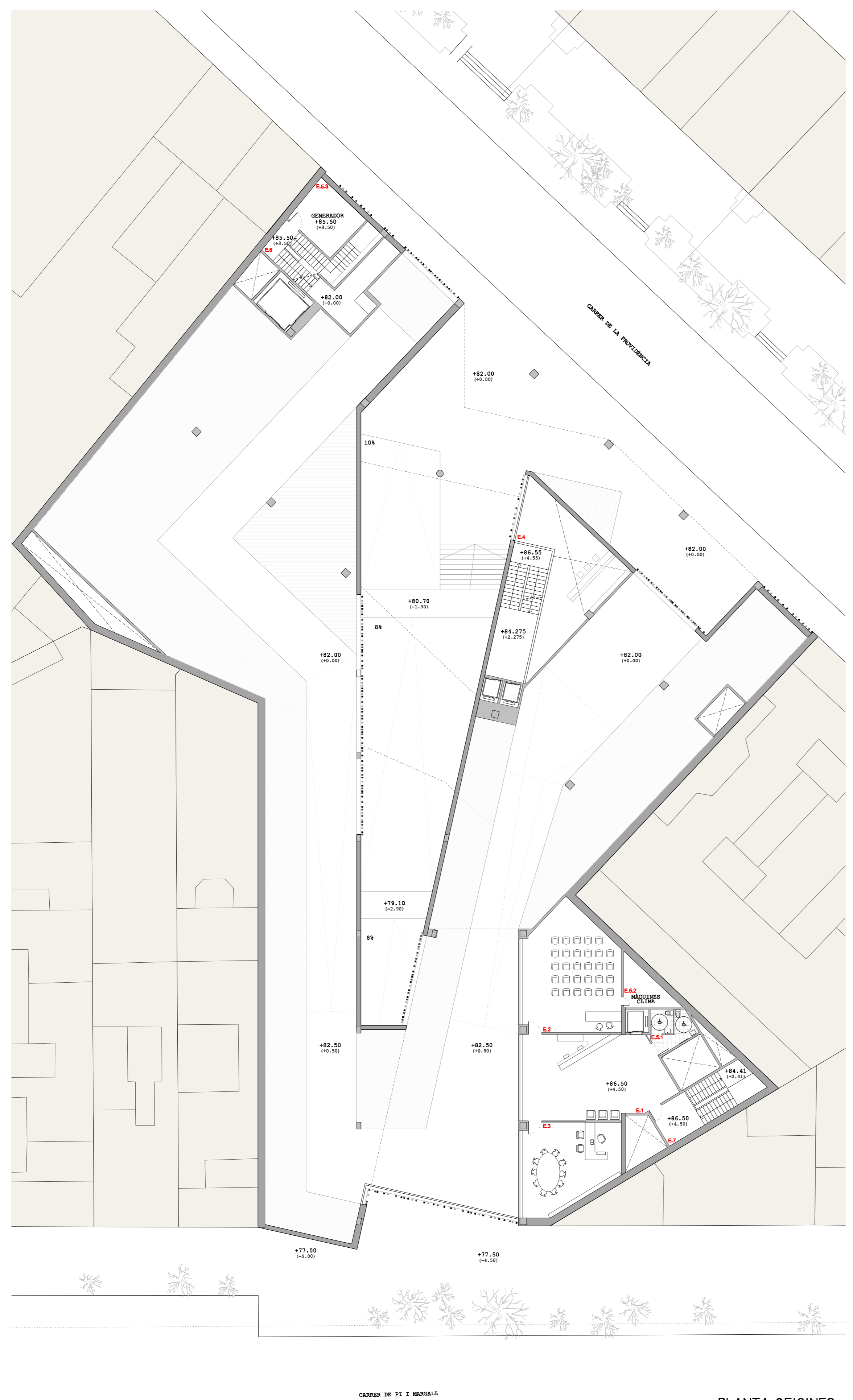
PLANTA OFICINES
