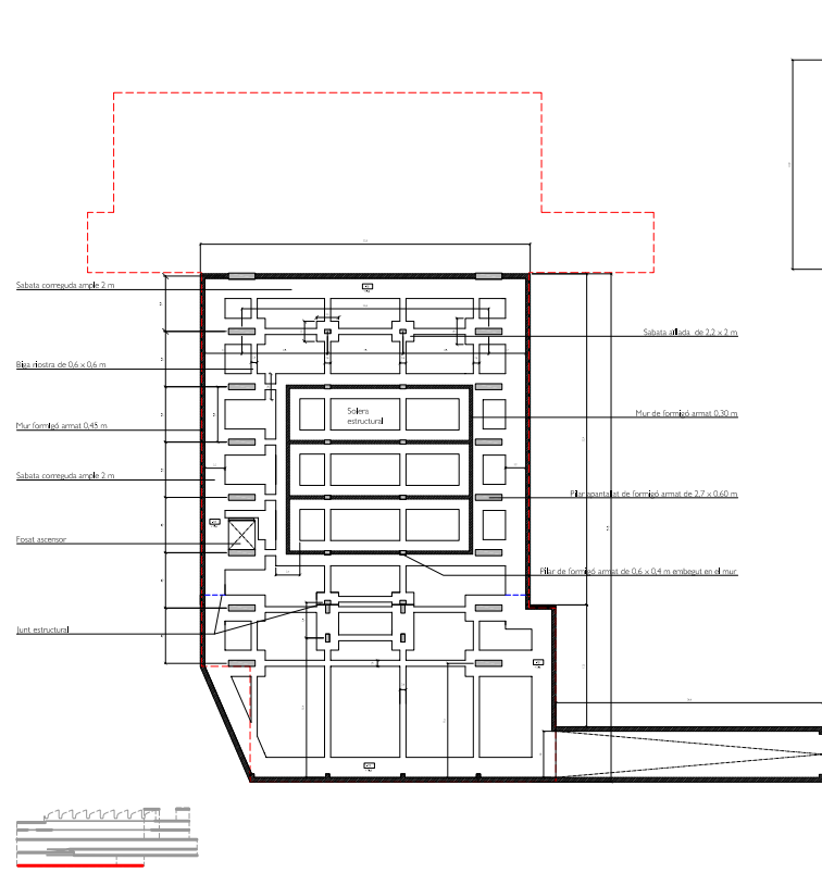
Planta fonaments (Planta residus)
