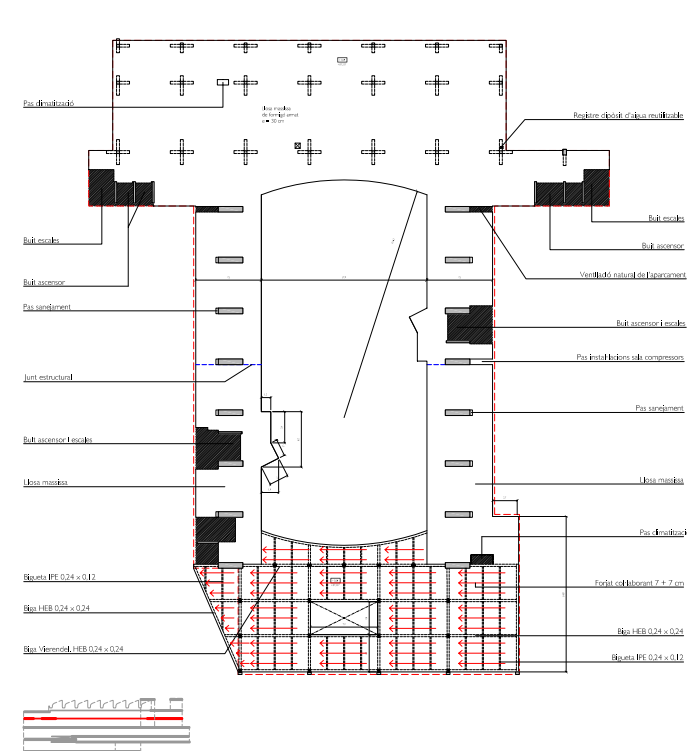
Forjat planta primera (Administració) 1.827 m 2
