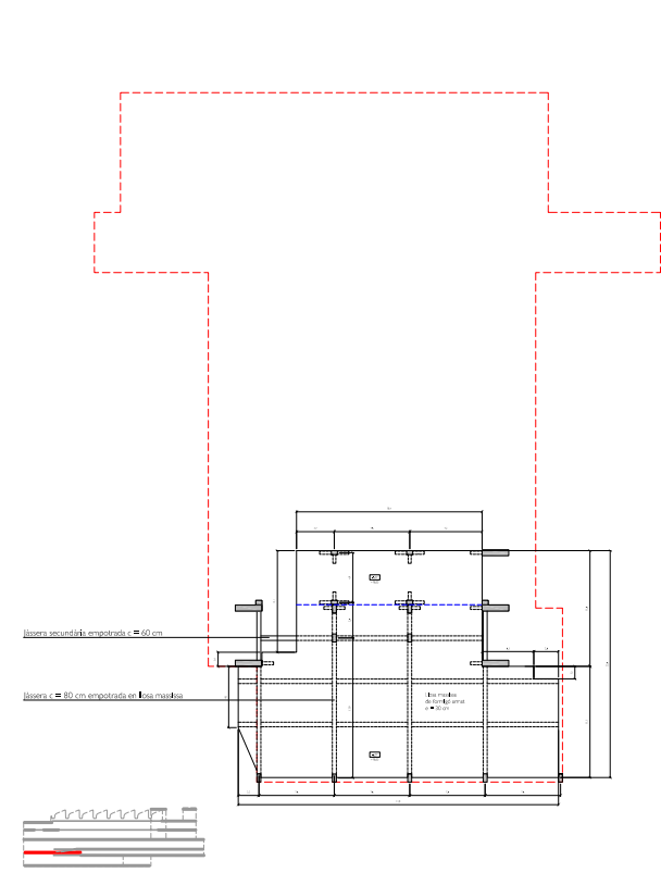
Forjat planta soterrani -1B (Càrrega i descàrrega) 560 m 2
