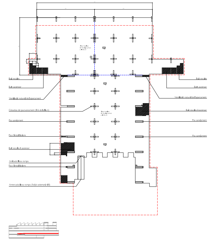
Forjat planta soterrani -1A (Magatzems) 2.050 m 2
