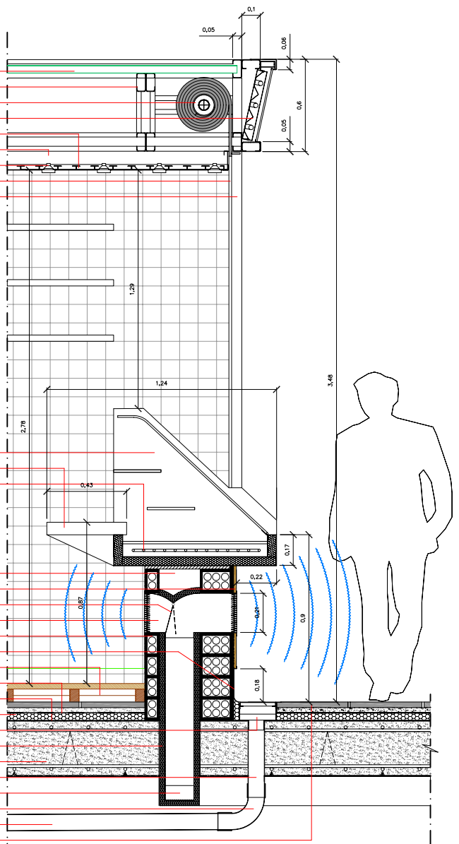
secció constructiva
