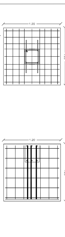
ARMADURA DE MUNTATGE D'ÀBAC CENTRAL AMB PILAR DE FORMIGÓ
