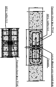
JUNTA AMB PASSADORS TITAN e 1/20
