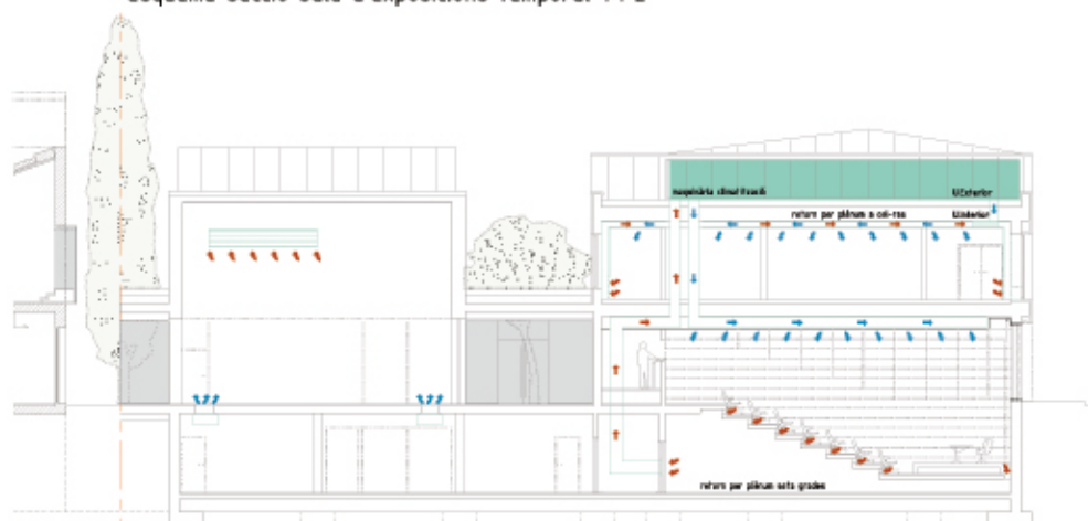
esquema secció sala de conferències i sala d'exposicions temporal 2
