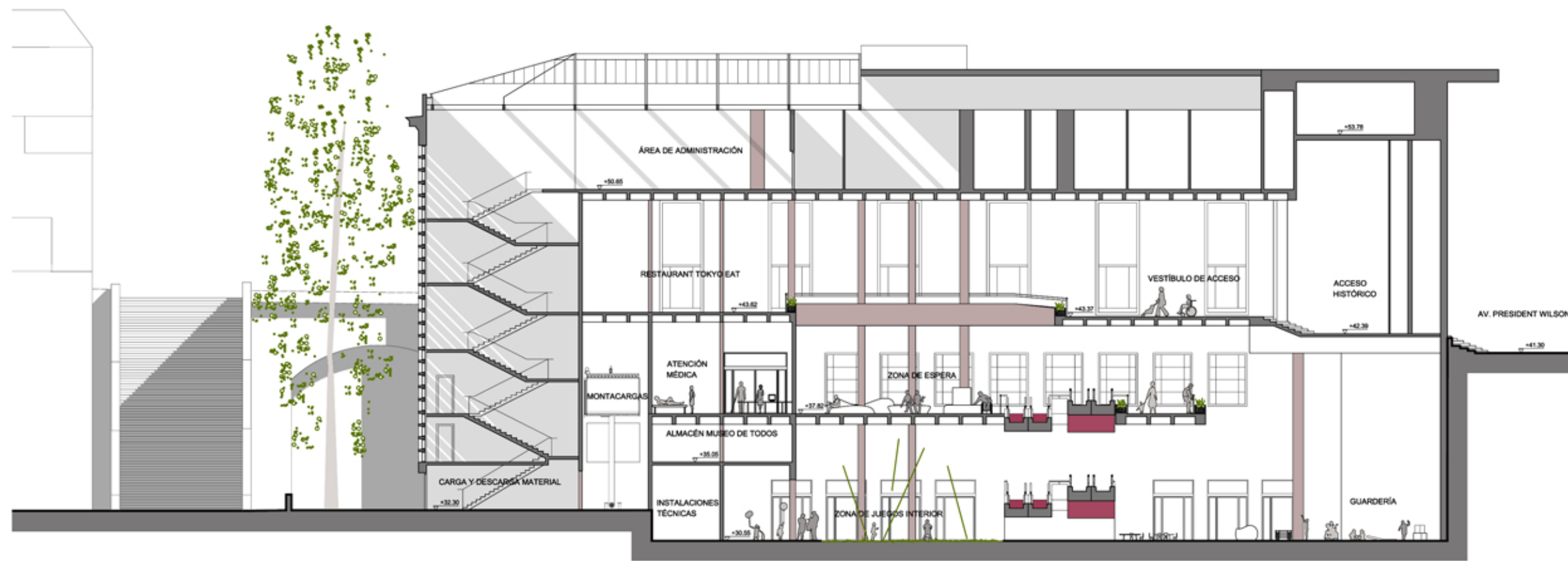
SECCIÓN A-A'
