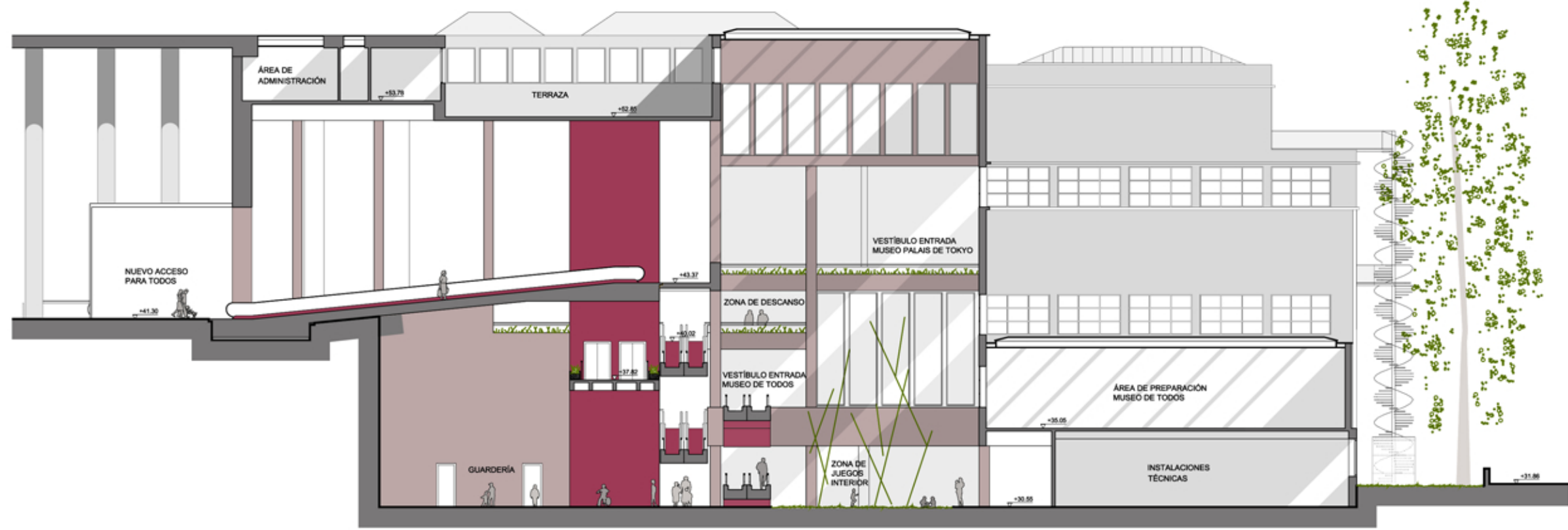
SECCIÓN B-B'
