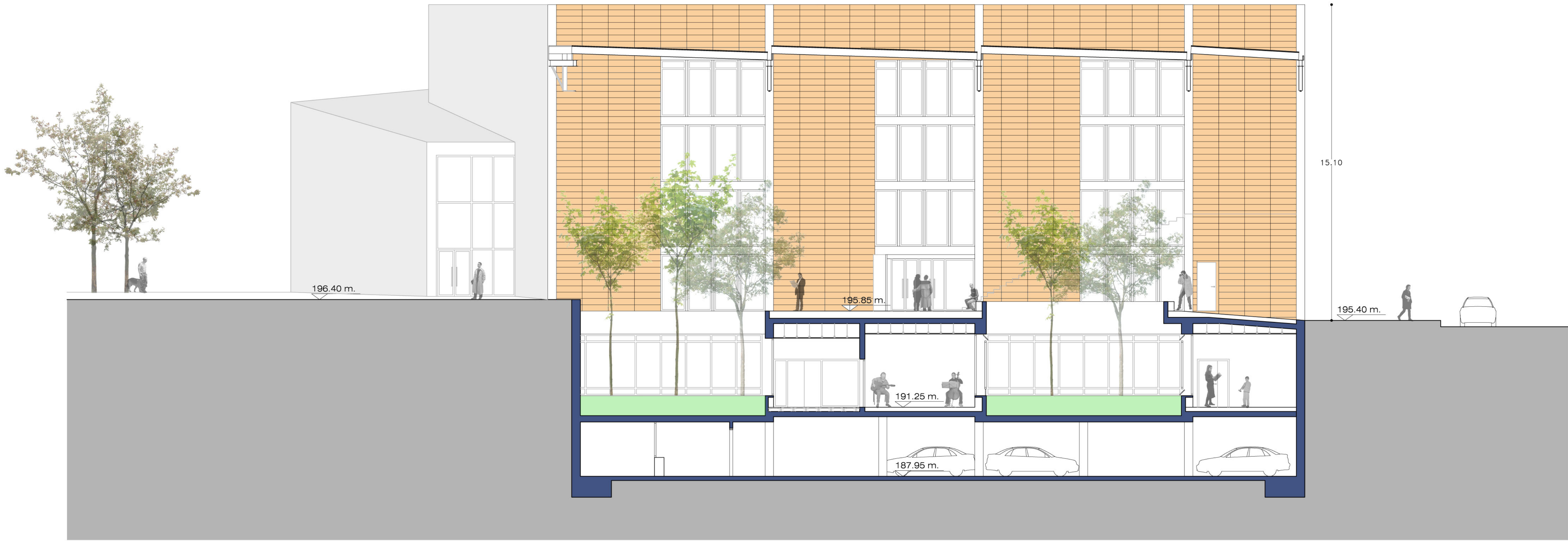
SECCION C - C'
