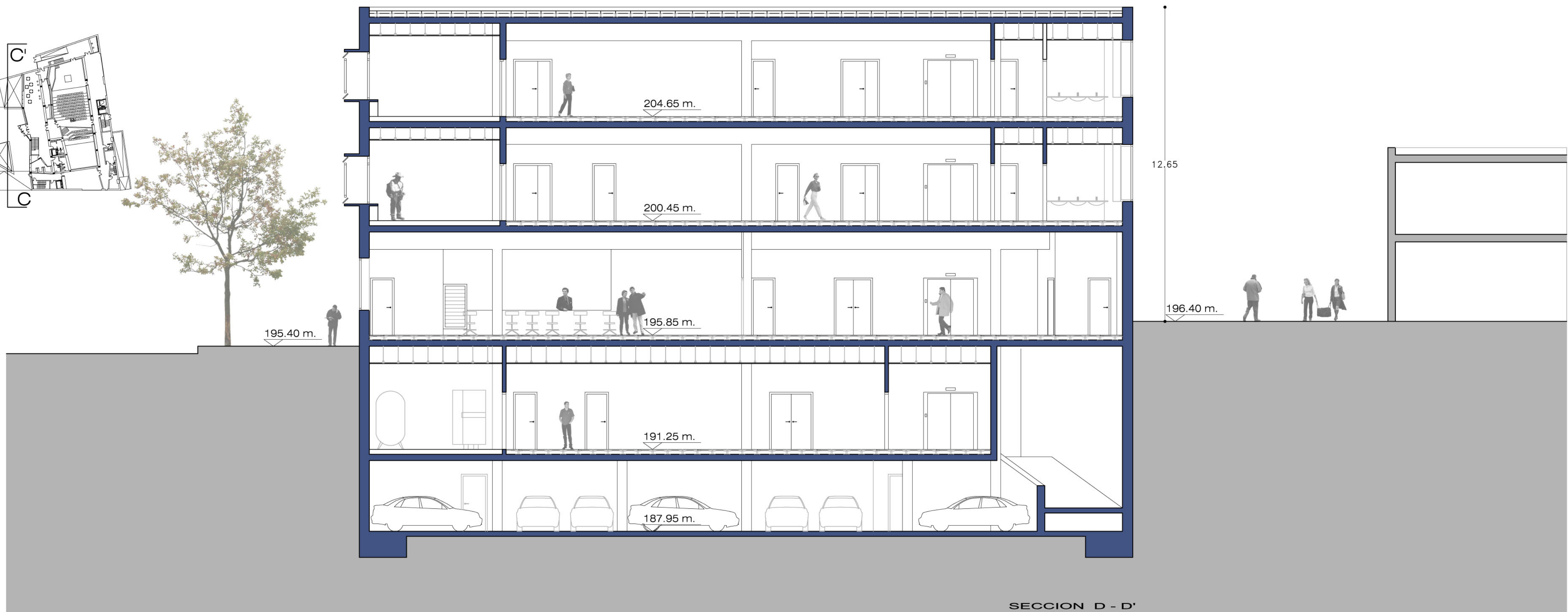
SECCION D - D'
