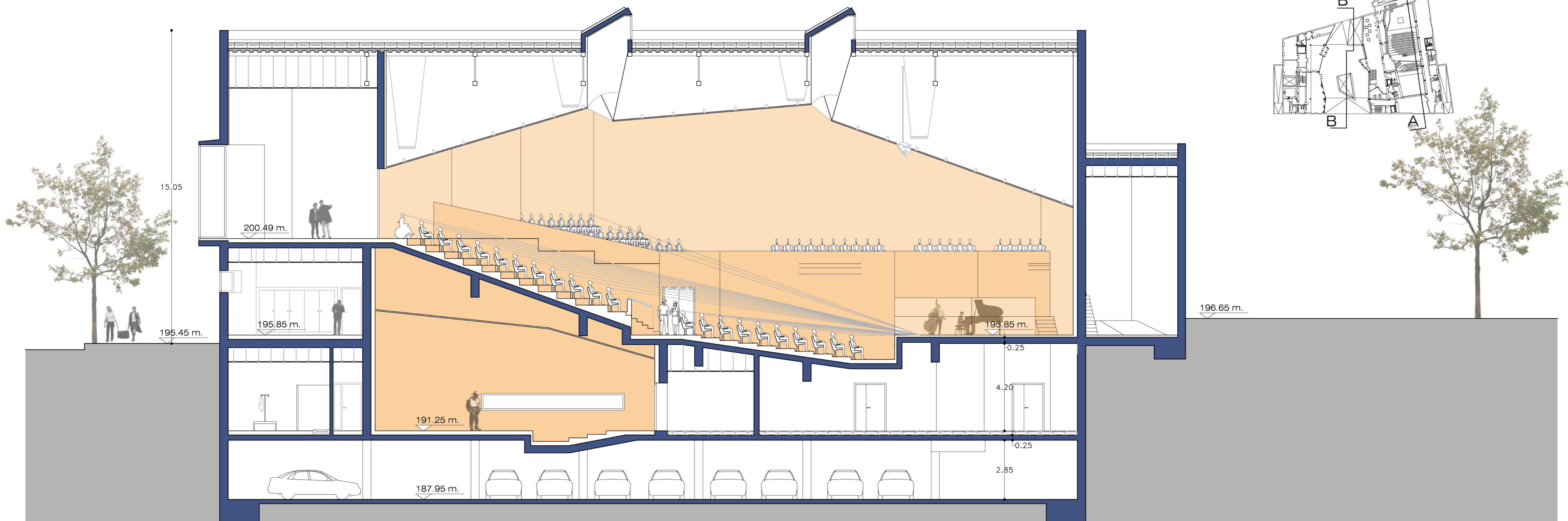
SECCION A - A'
