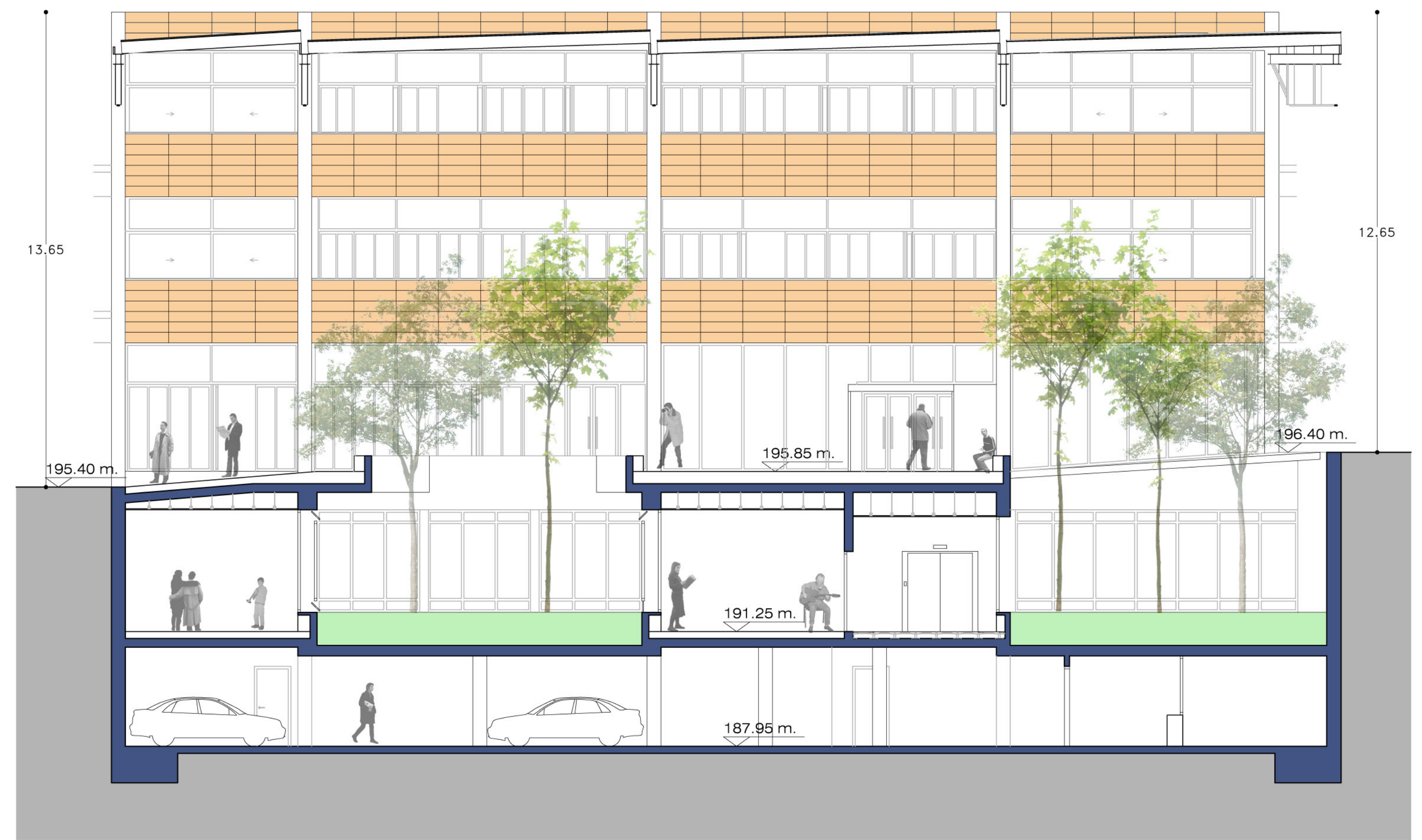
SECCION B - B'
