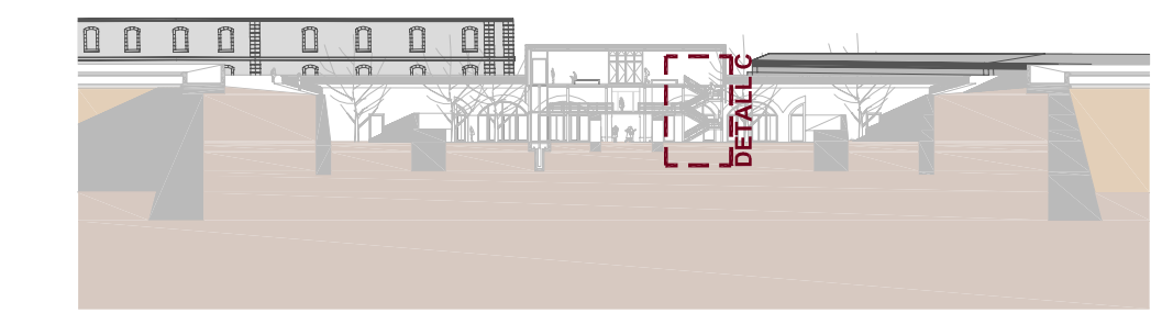
D_02 secció transversal mòdul escala e:1/15
