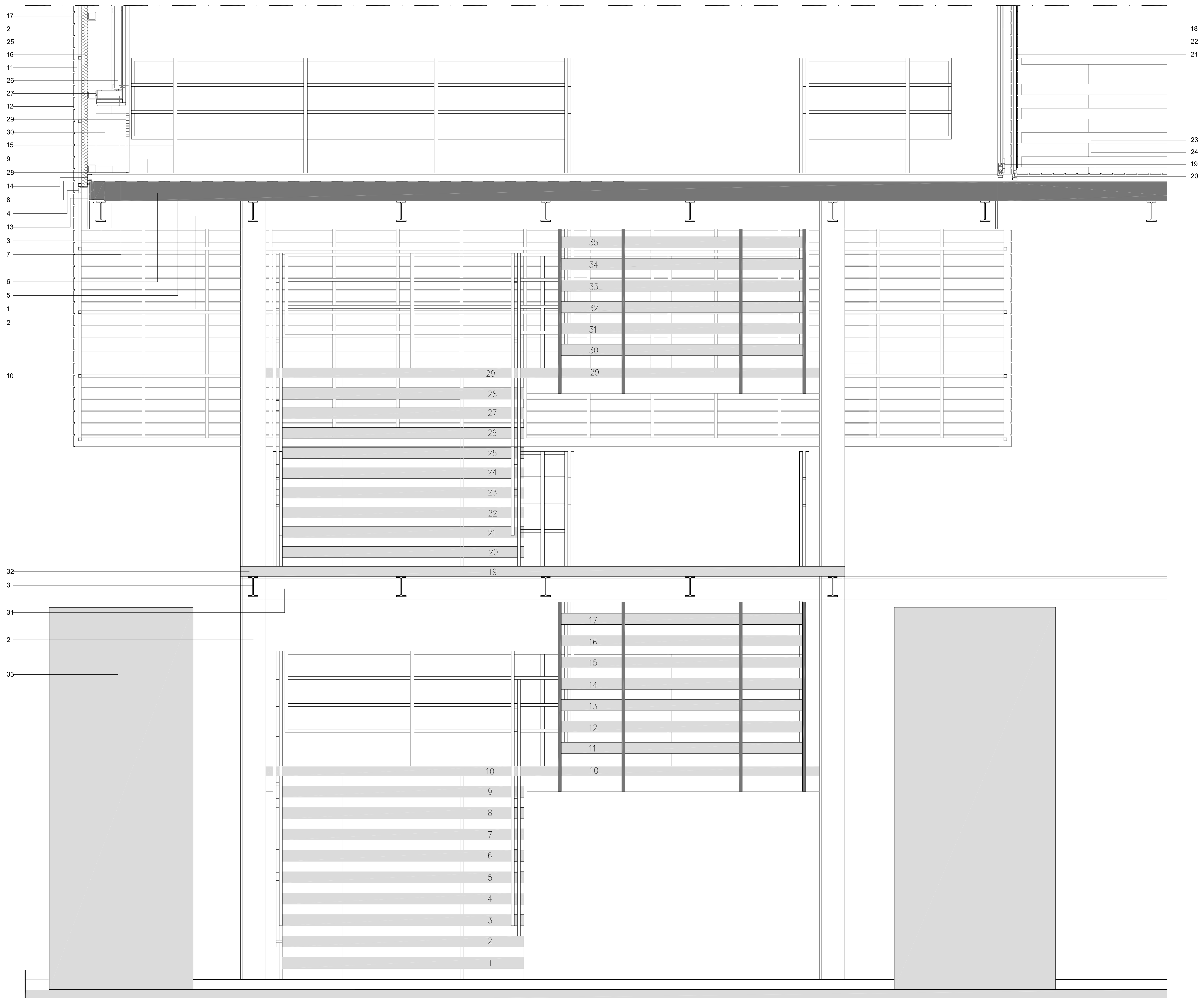
D_02 secció transversal mòdul escala e:1/15
