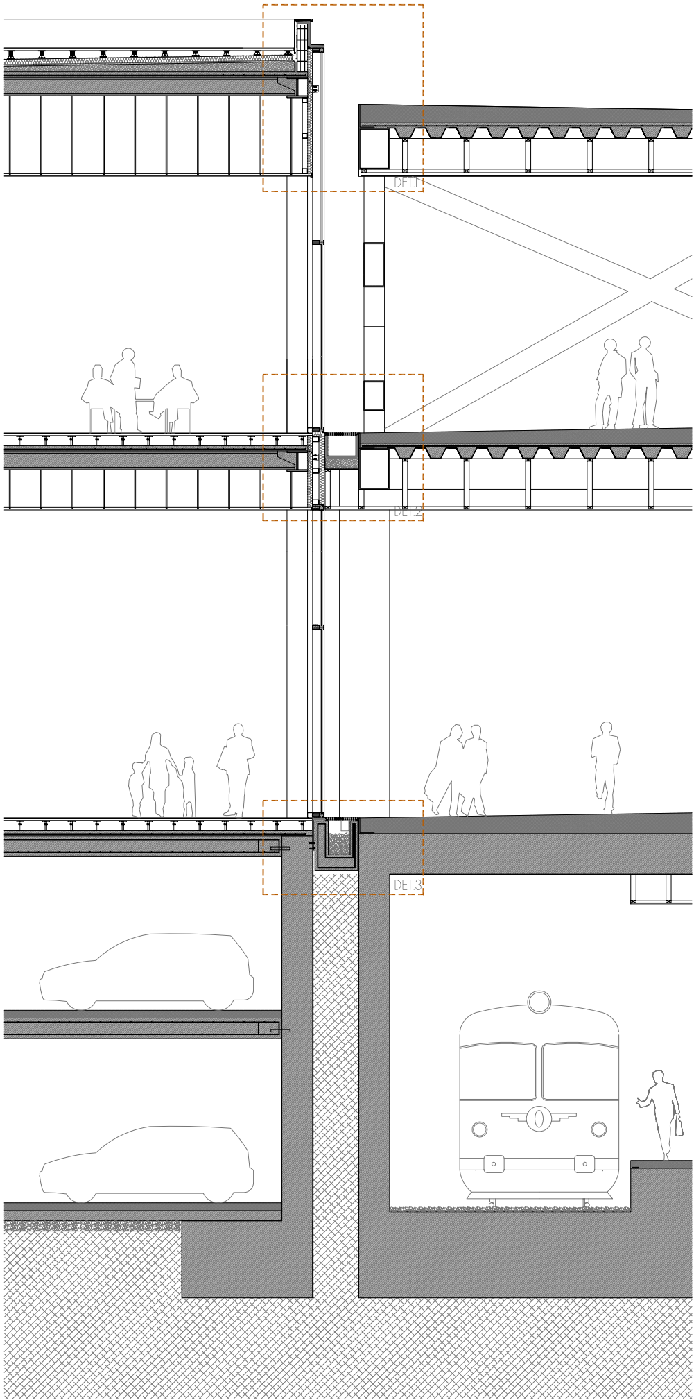
SECCIÓ VERTICAL ENCONTRE EDIFICI I PASSERA
