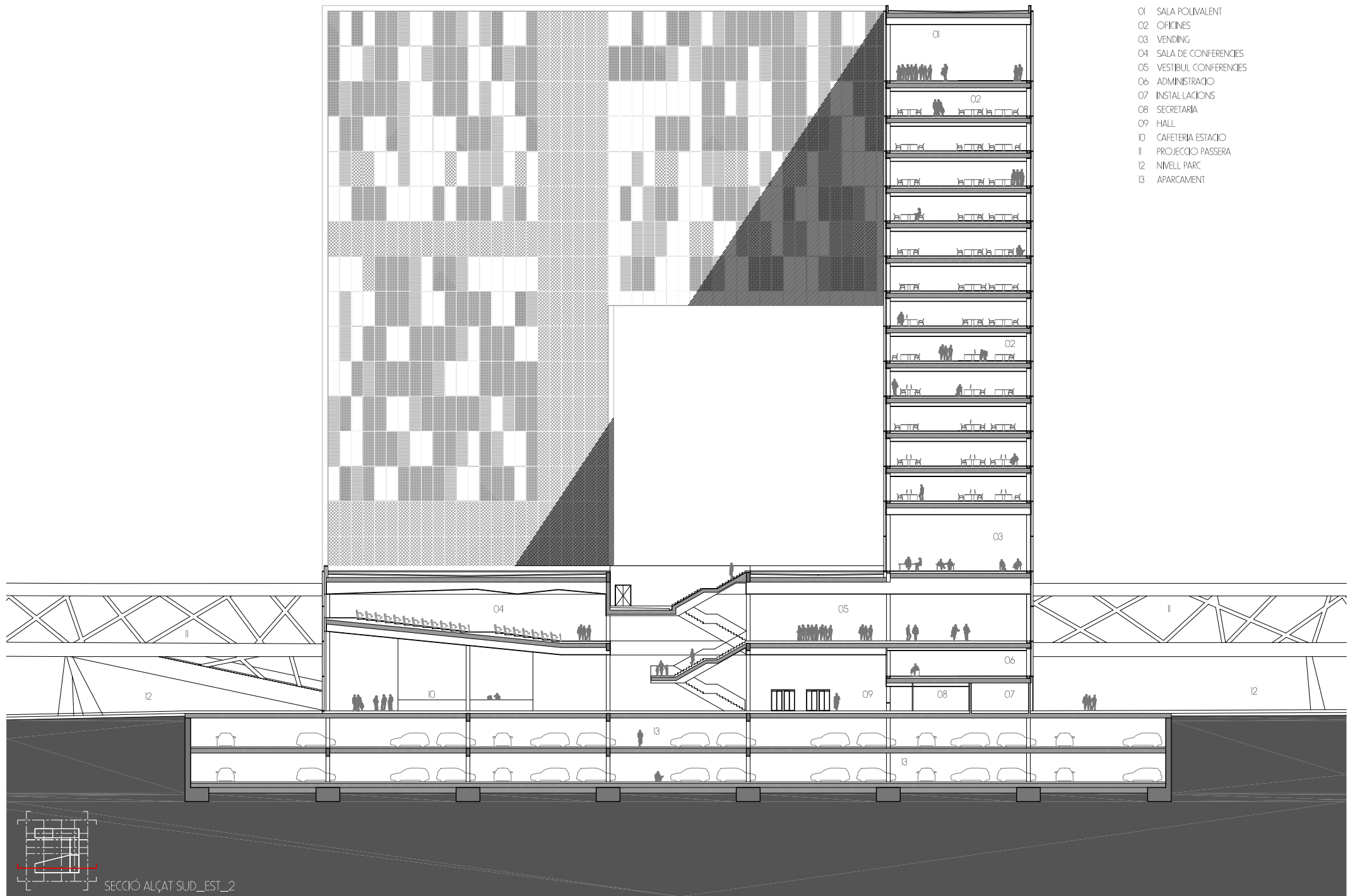
SECCIÓ ALÇAT SUD_EST_2
