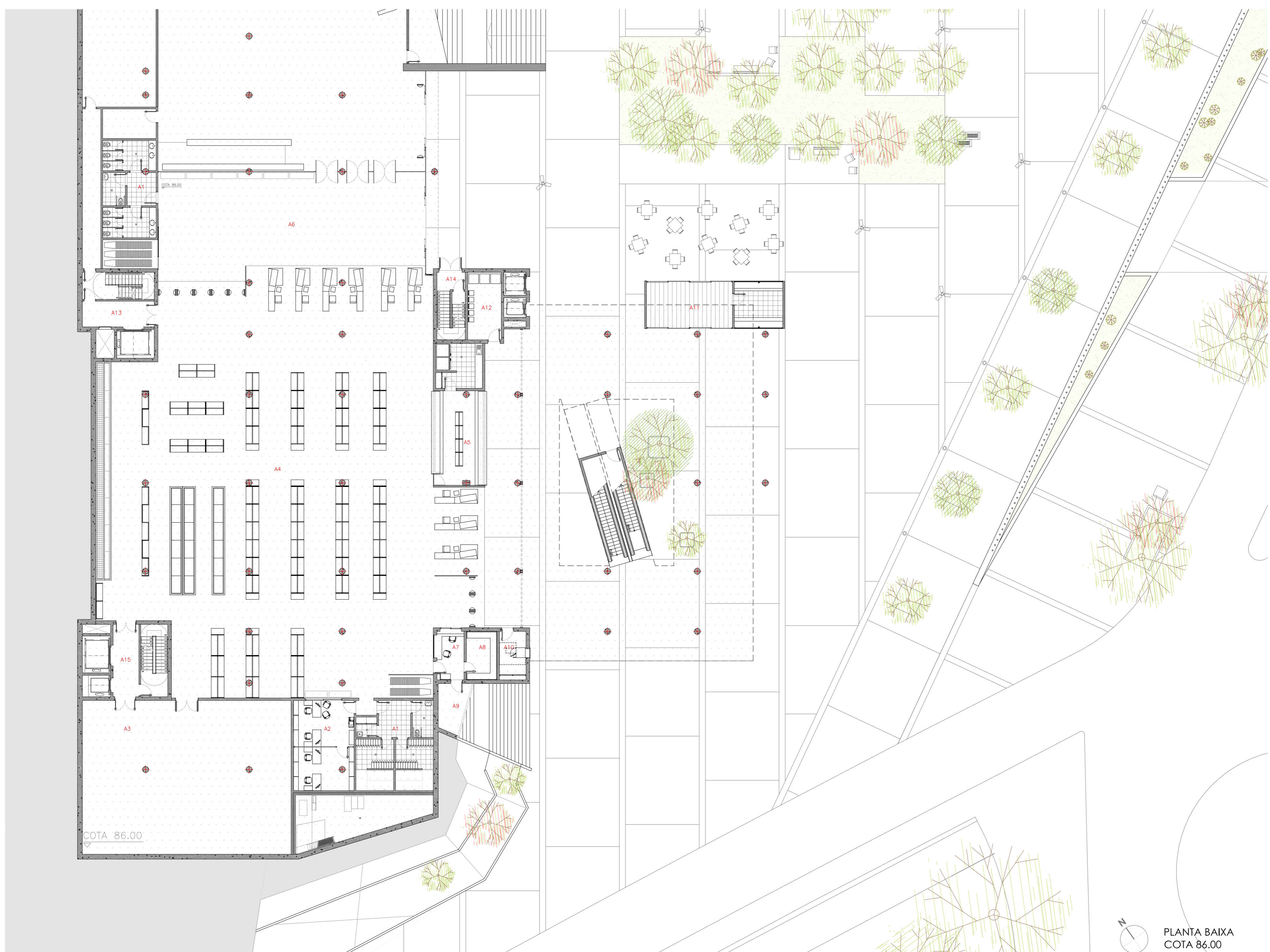
PLANTA MERCAT COTA 90.50
