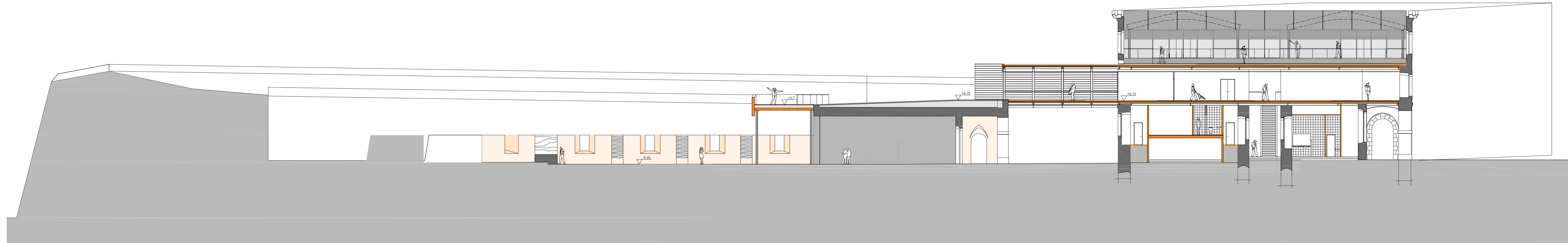
SECCIÓ TRANSVERSAL B-B'
