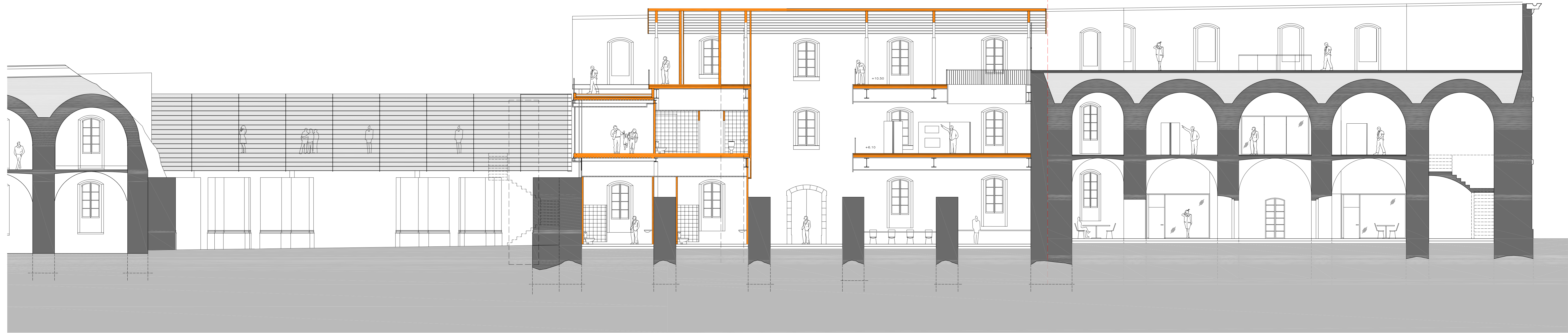
SECCIÓ LONGITUDINAL F-F
