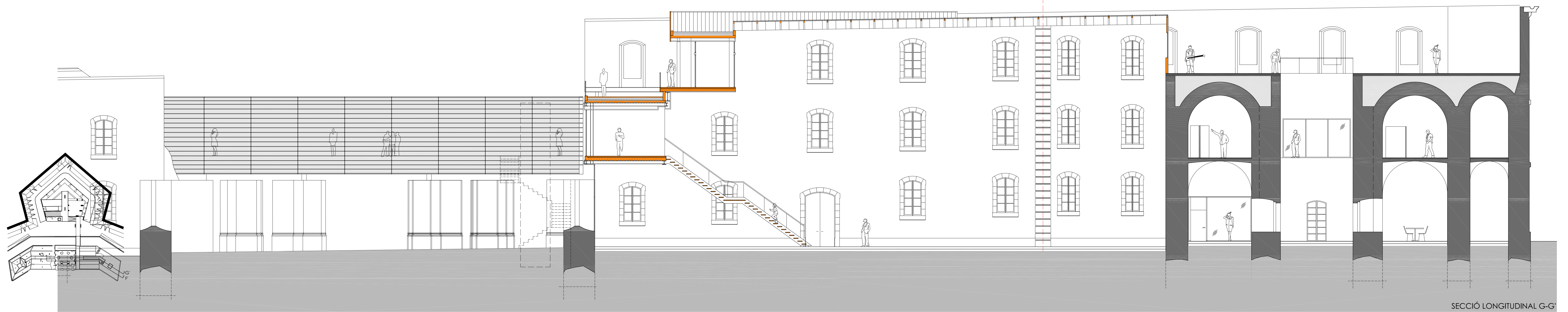
SECCIÓ LONGITUDINAL G-G
