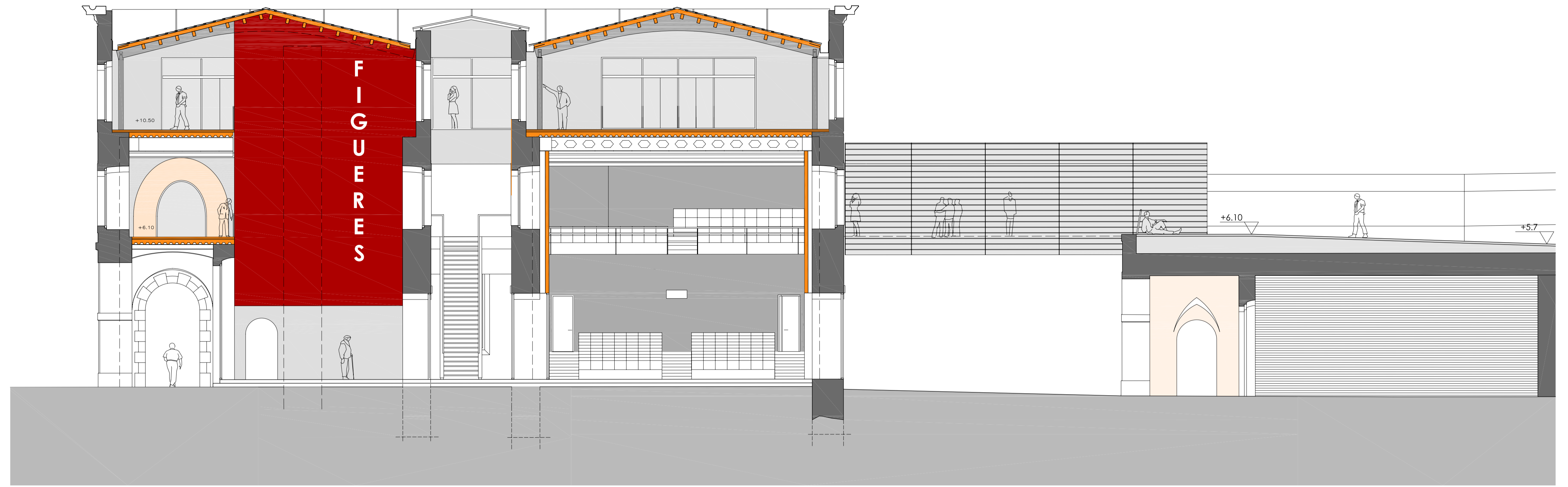
SECCIÓ LONGITUDINAL A-A'
