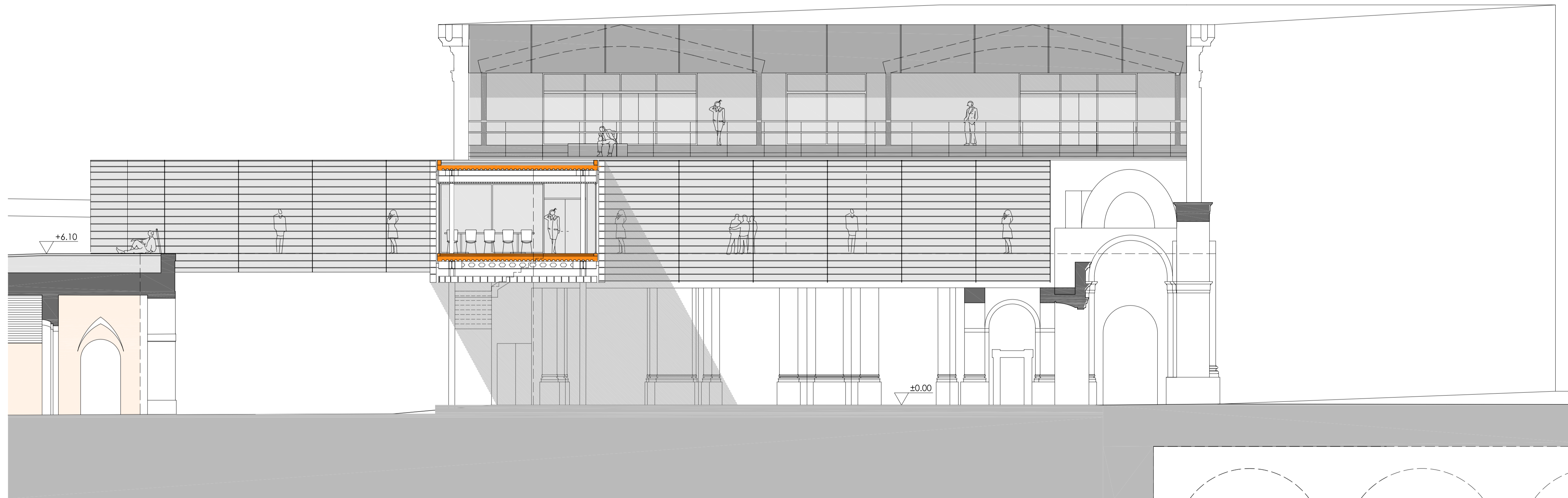
SECCIÓ LONGITUDINAL C-C'
