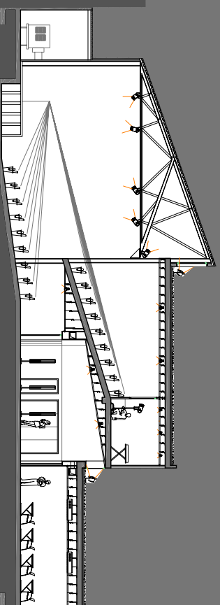
SECCIÓ E-E'
