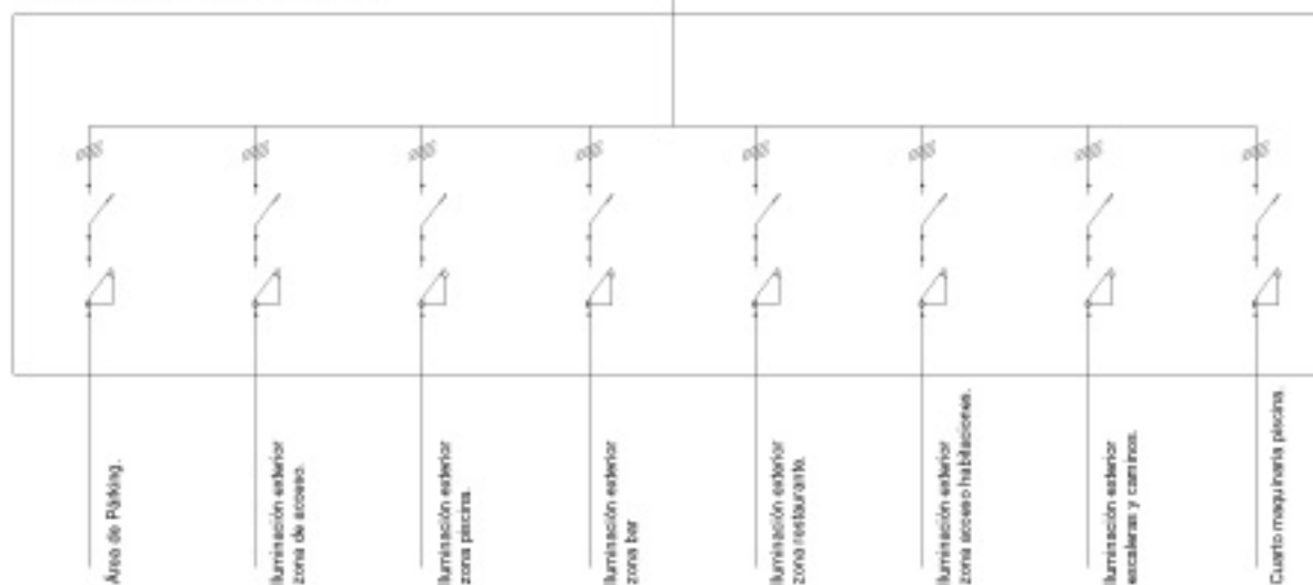
Cuadro Instalación Exterior.
