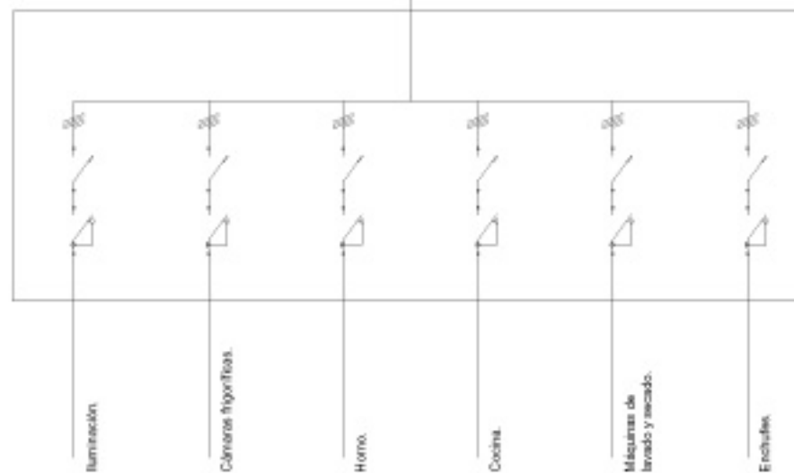
Subcuadro Cocina Restaurante.
