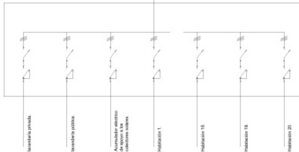
Cuadro Edificio Residencial.
