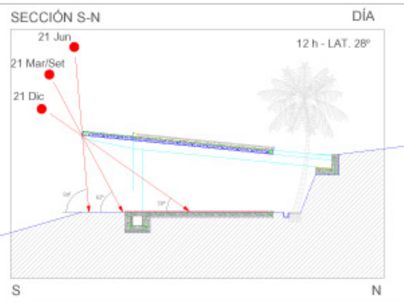
Protección horizontal: alero fijo.
