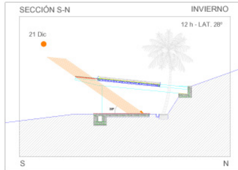
Protección horizontal: lamas móviles.
