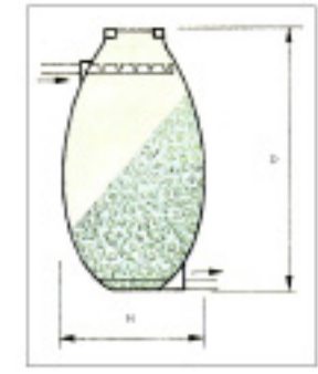
Filtro biológico de material plástico
