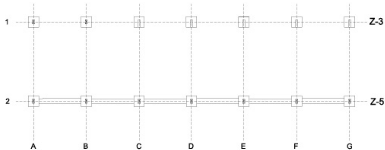
Planta de Cimentación - Edificio Restaurante. (3)
