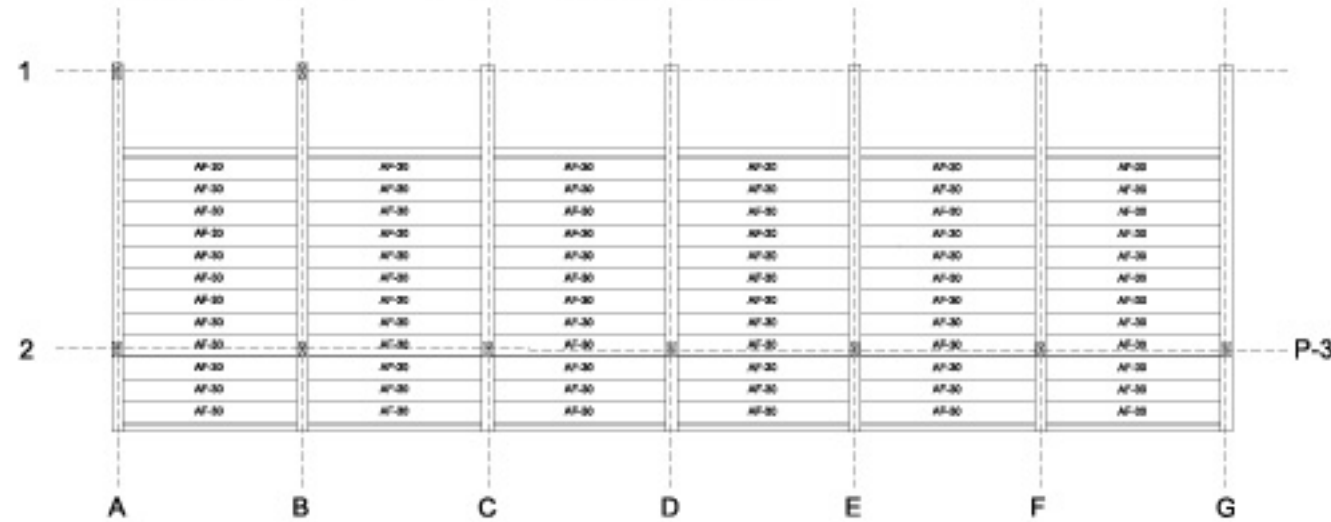
Forjado de techo - Edificio Restaurante. (3)
