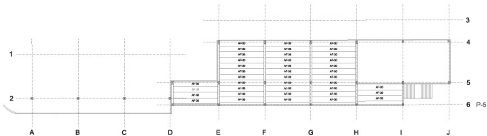
Forjado de techo - Edificio Edificio Almacén - Planta Baja.
