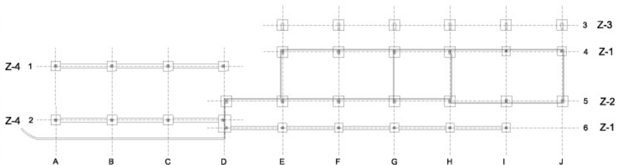
Planta de Cimentación - Edificio Recepción y Almacén.
