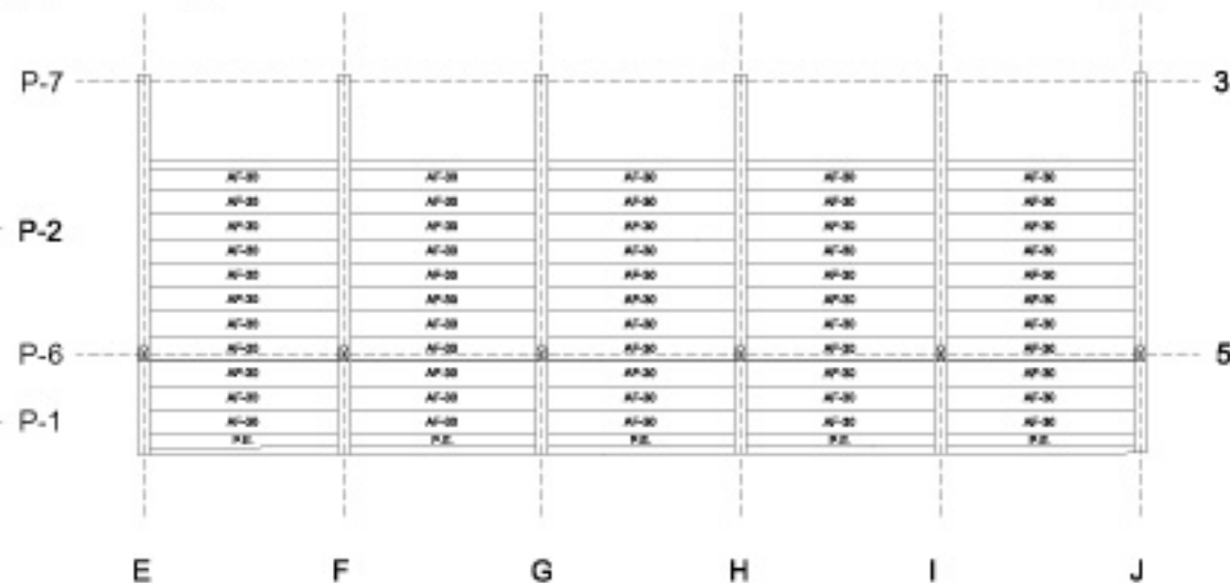
Forjado de techo - Edificio Edificio Almacén - Planta 1. (2)
