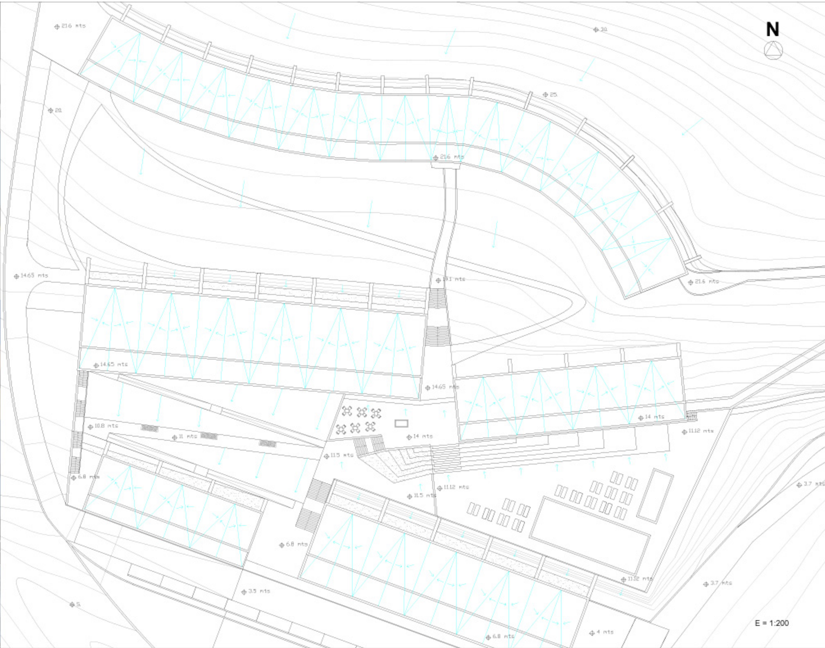
P 12. Planta de Cubiertas. Centro Internacional para Windsurfistas en Playa de Vargas - Gran Canaria.
