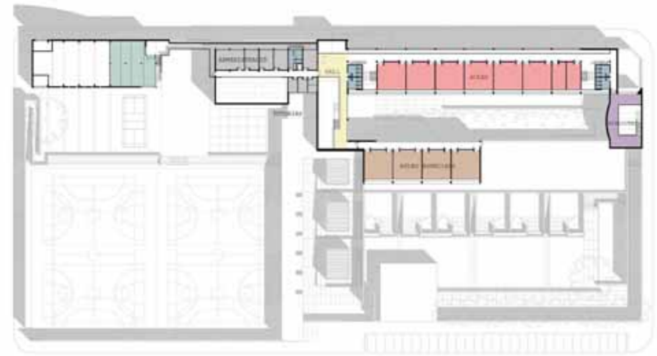
PROGRAMA FUNCIONAL PLANTA PRIMERA
