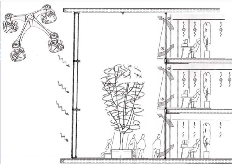
DETALL MUR CORTINA EN ANCLATGES TIPUS ARANYA EN ZONA VERDA COMUNITÀRIA
