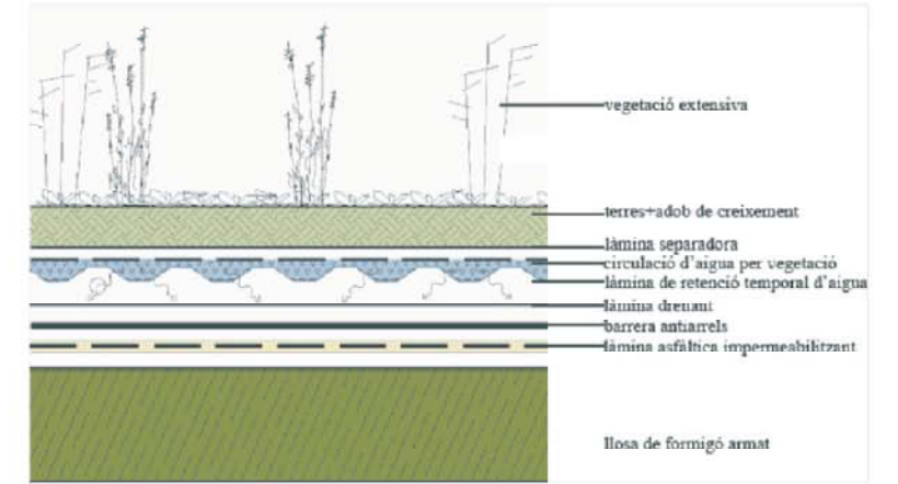
DETALL ZONA AJARDINADA DELS ESPAIS COMUNITARIS PER PLANTACIÓ EXTENSIVA PER SISTEMA DE REGAT CONTÍNU INTEGRAT EN PLATAFORMA INFERIOR
